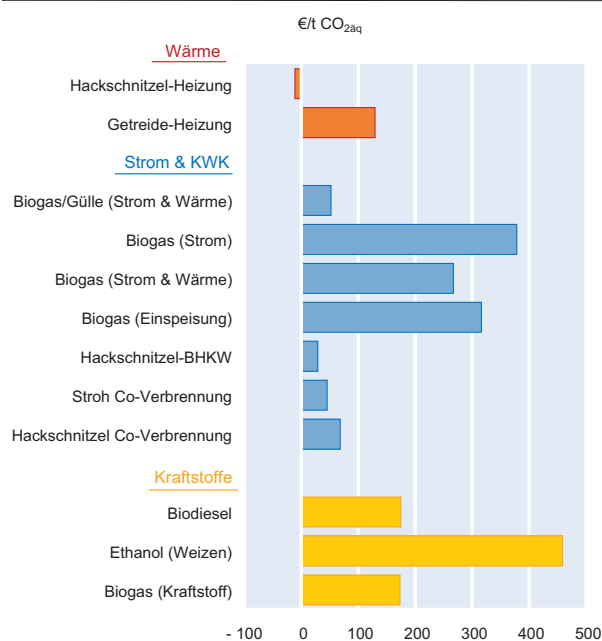
Abb. 3 CO 2äq -Vermeidungskosten verschiedener Bioenergielinien
