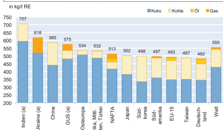
Abb. 3 Reduktionsmittelverbrauch der Hochöfen weltweit, 2005
