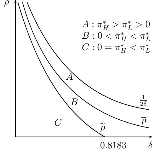
Figure 1 : Parameter Space
