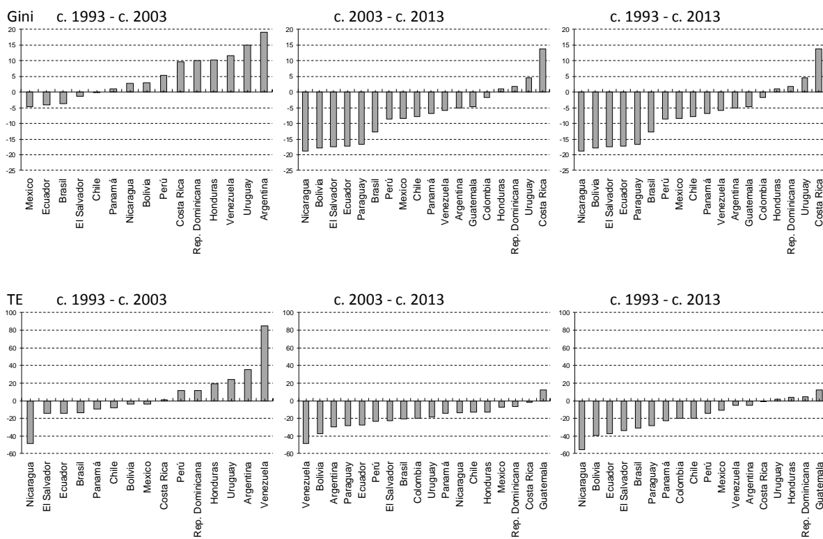
Figura 4.6: Cambio % en el coeficiente de Gini y Tasa de Extracción
