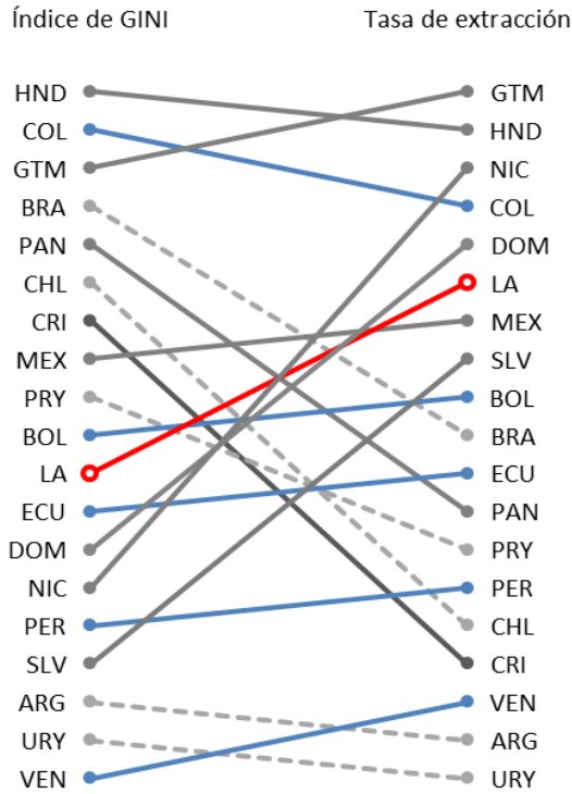
Figura 4.4: Cambio de rankings según diferentes medidas de desigualdad. Países de América Latina. Circa 2013.
