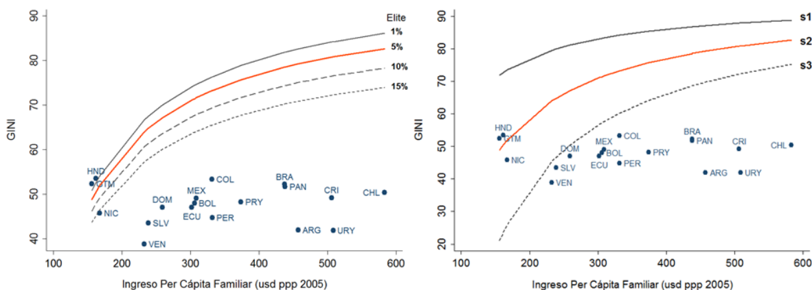
Figura 4.2: Frontera de posibilidades de desigualdad. Países de América Latina. Circa 2013.
