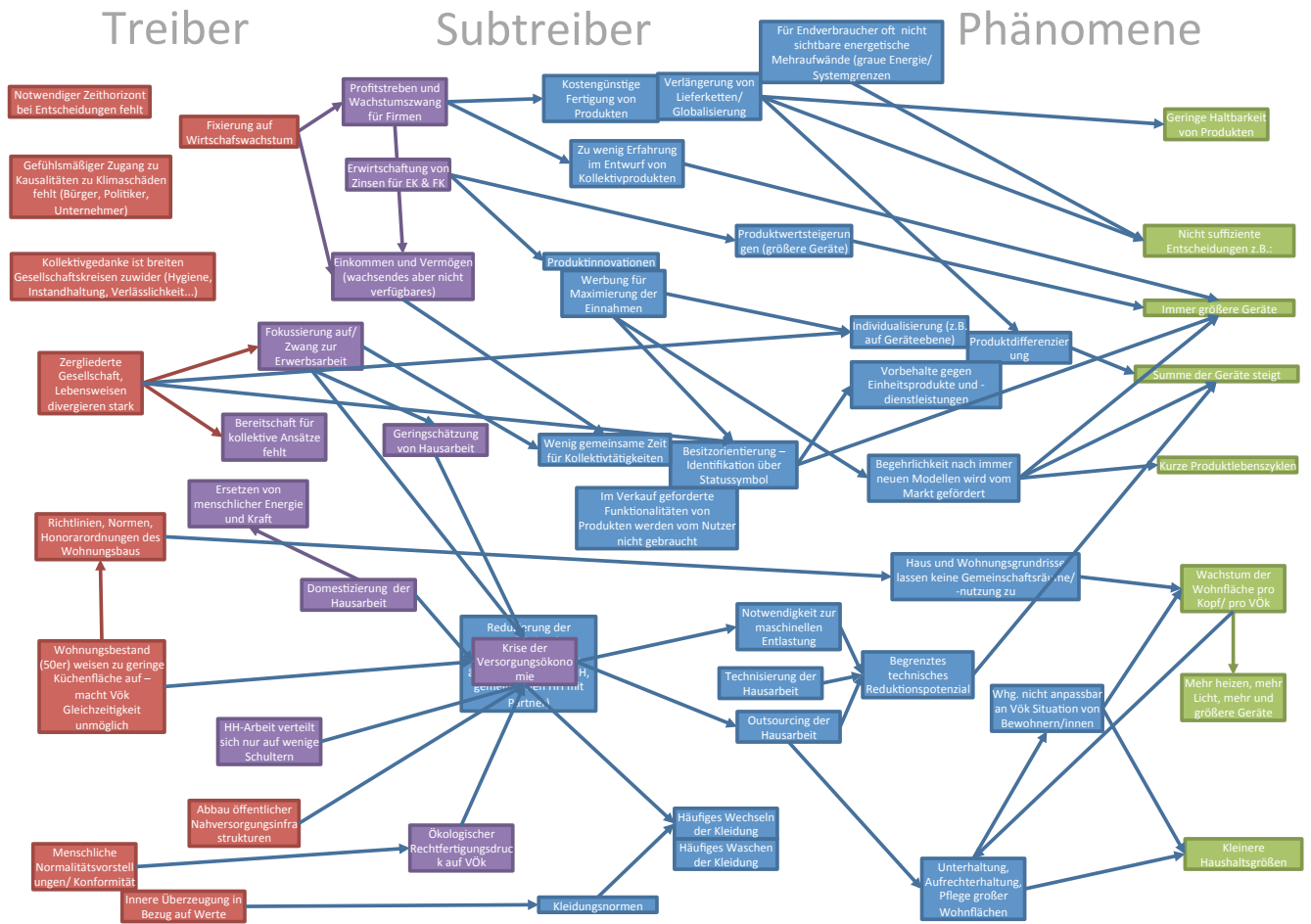
Abbildung 7: Einordnung in Treiber, Subtreiber und Phänomene der Nicht-Energiesuffizienz
