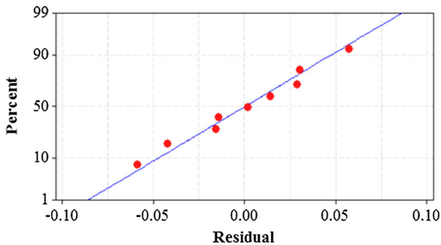
Fig. 5 Curvilinear model: actual values versus predicted values of SR
