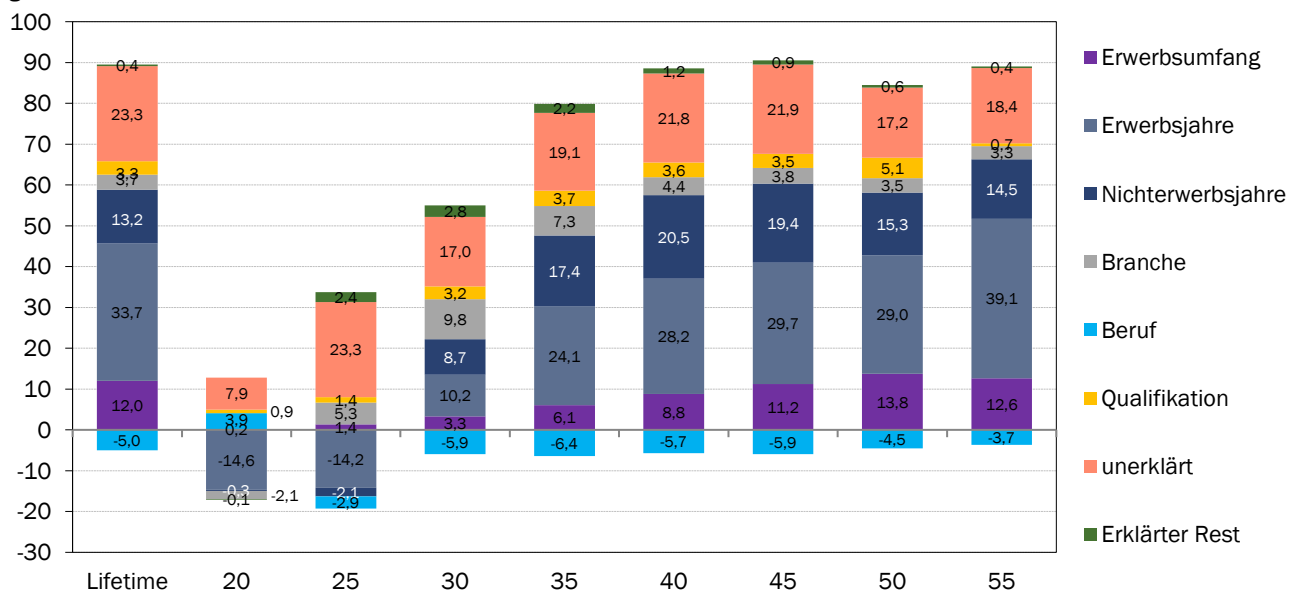
Abbildung 25: Haupteinflussfaktoren des erklärten Teils des Gender Earnings Gap nach Alter
