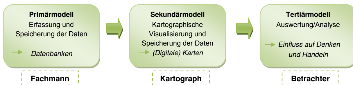
Abbildung 5: Kartographisches Kommunikationsmodell
