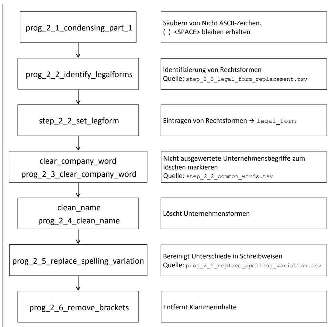
Abbildung 4: Ablaufplan: Funktionen Routinen der Stufe 2.
