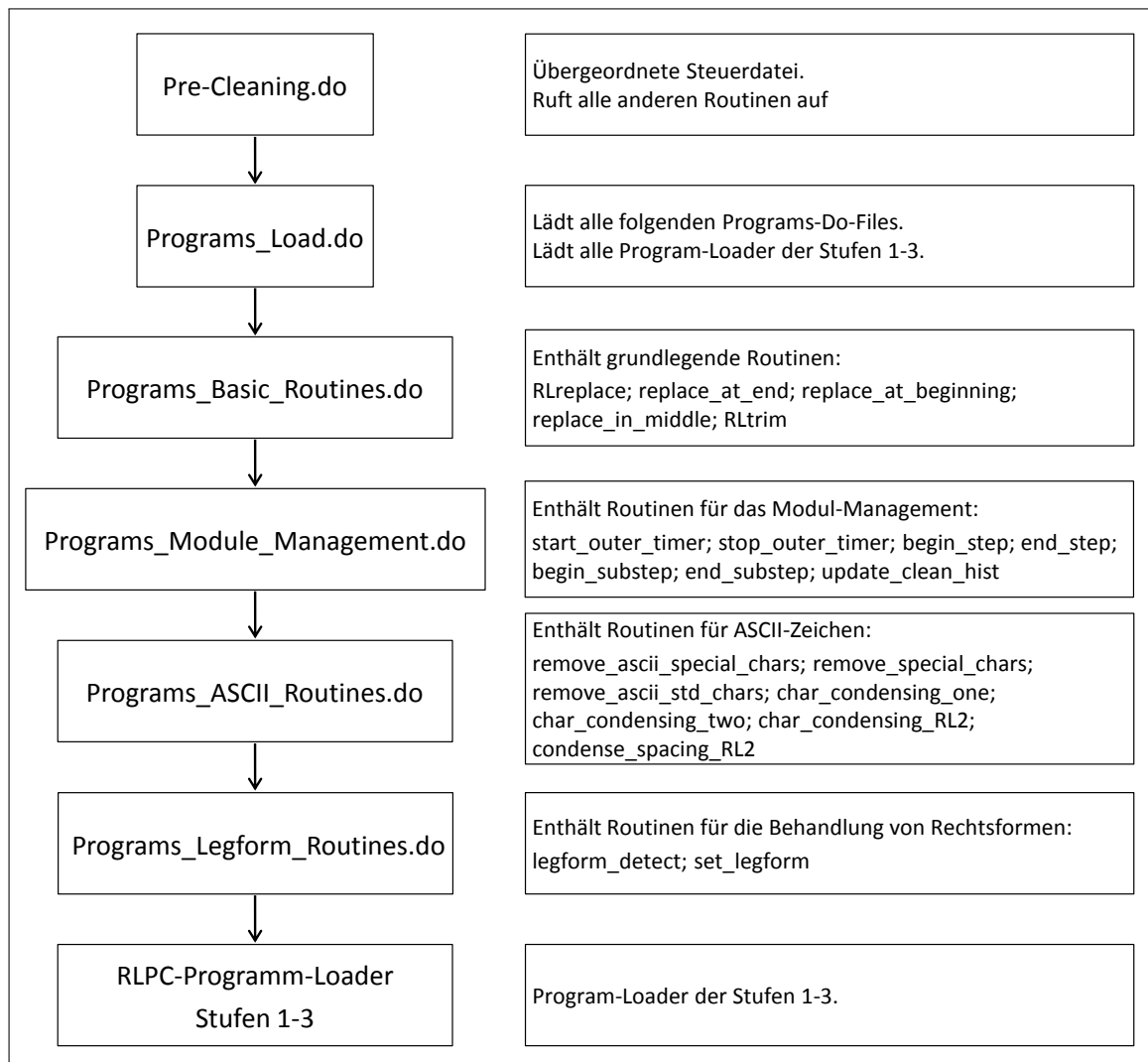
Abbildung 2: Ablaufplan: Laden der grundlegenden Routinen.
