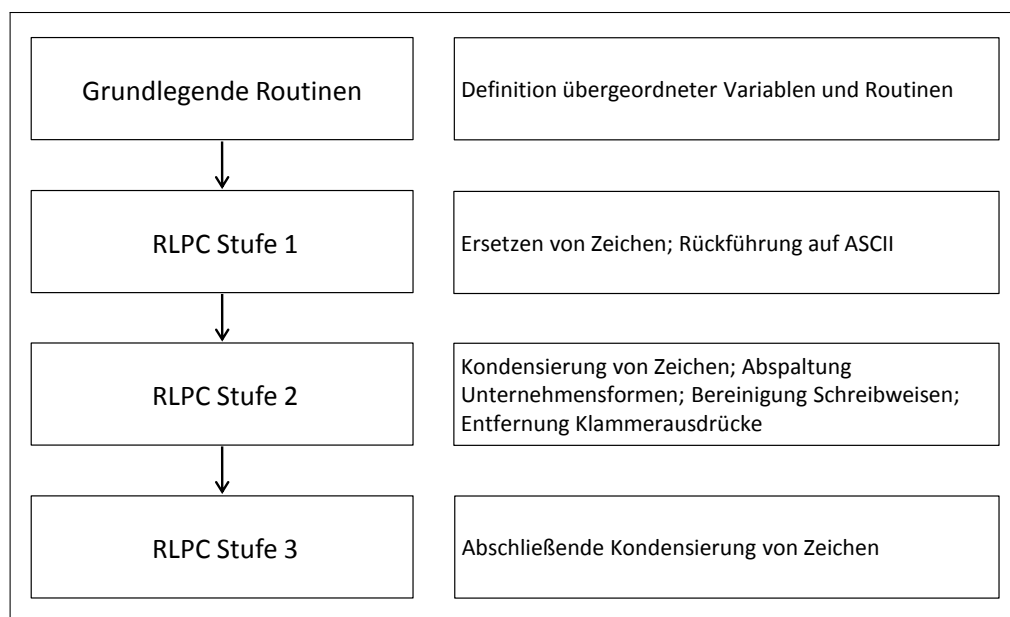
Abbildung 1: Ablaufplan: Struktureller Ablauf des Verfahrens in Stufen.
