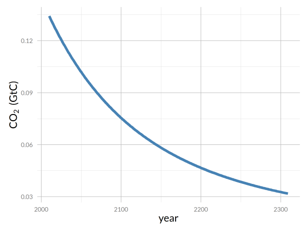
(d) CO_2 Emissions
