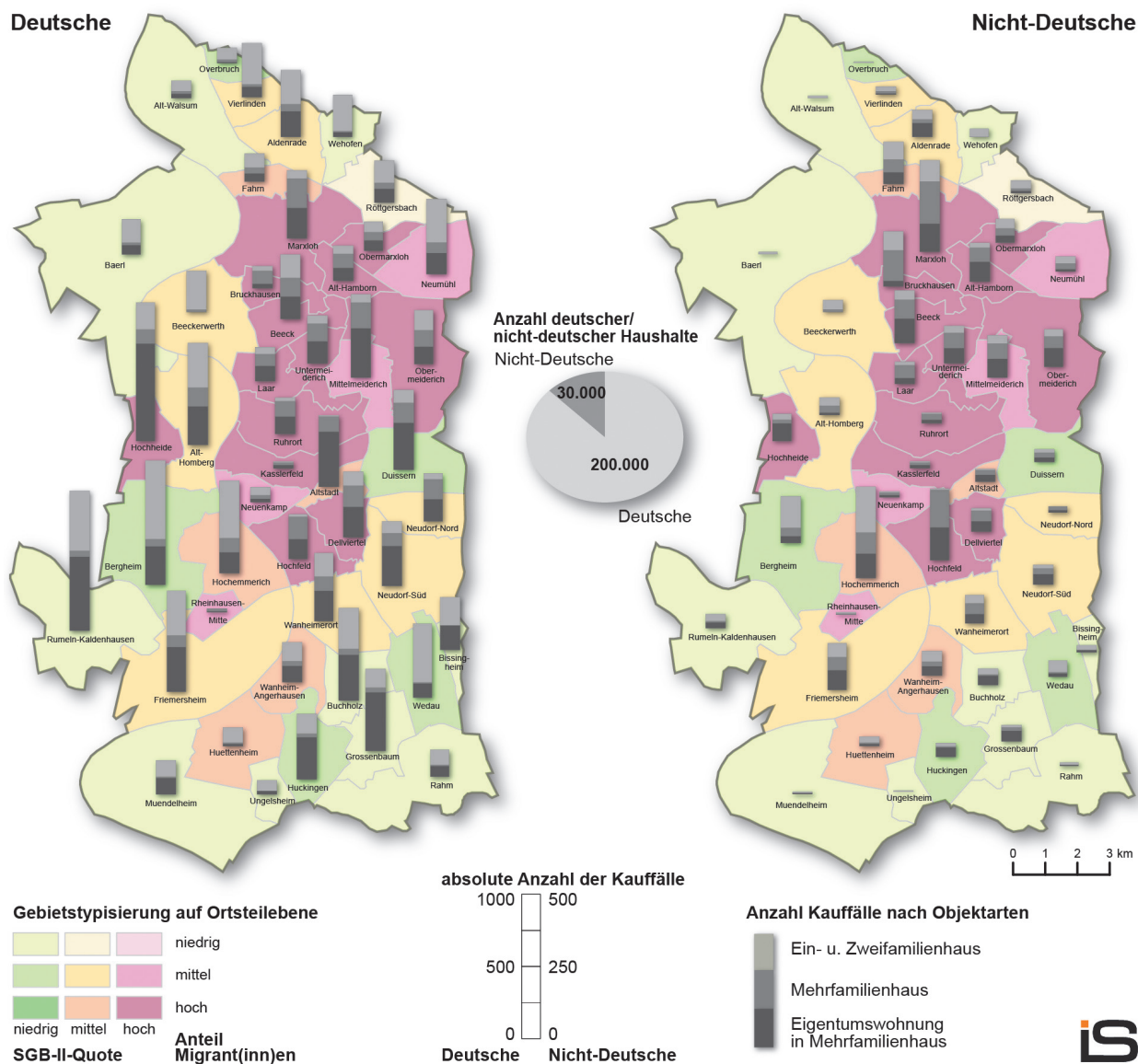
Abb. 2: Deutsche und nicht-deutsche Käufer(innen) in der Stadt Duisburg (1998 – 2006)
