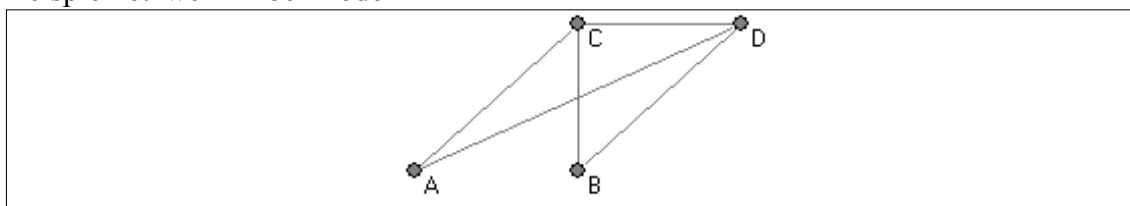
Abbildung 2: Beispielnetzwerk Blockmodell
