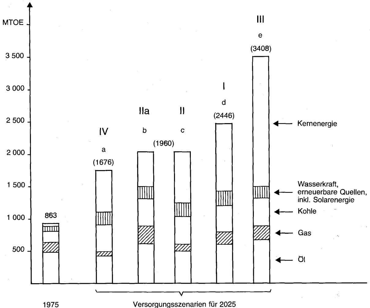
Abbildung 1 Primärenergieeinsatz in der EG im Jahre 1975 und im Jahre 2025 nach den fünf Szenarien
