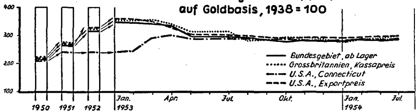
Prozentuale Entwicklung der Zinnpreise auf Goldbasis, 1938 = 100
