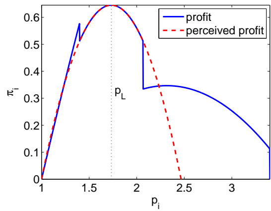
(d) Profit functions of low-price firms (ALE)
