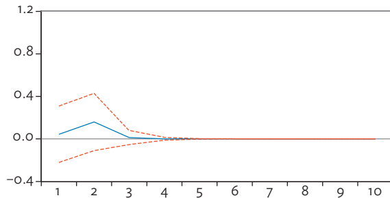
Response of D (AUS_GINI) to D (AUS_LGDPC)
