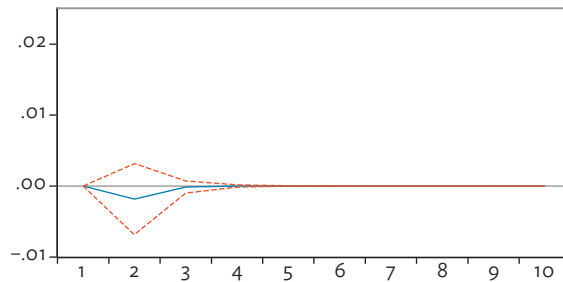
Response of D (AUS_GINI) to D (AUS_GINI)
