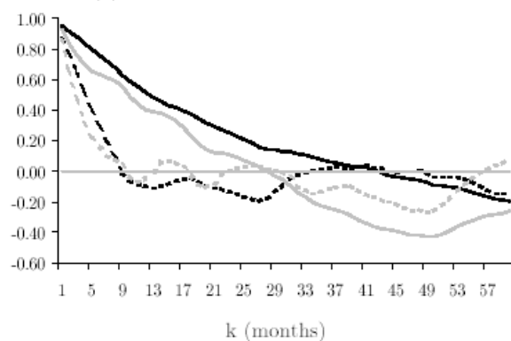
(d) Autocorrelation Coefficients: TERM
