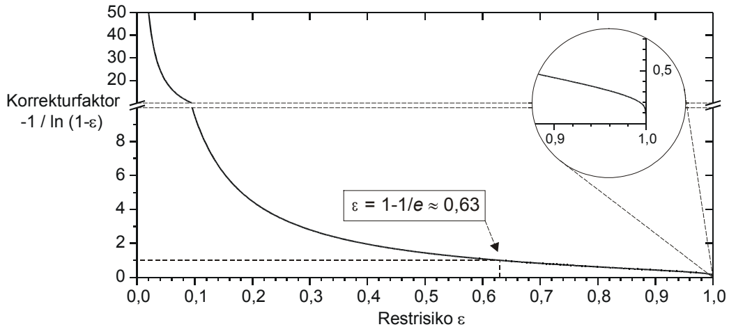
Abbildung 2: Korrekturfaktor für die Vergleichszeitdauer, die die mittlere Lebenszeit einer betrachteten Population überschreiten muss, damit diese Population einen Bestand darstellt, dargestellt in Abhängigkeit des akzeptierten Restrisikos \varepsilon . Für \varepsilon = 1 - e^{-1} \approx 0,63 wird der Korrekturfaktor gerade gleich 1, d.h. die Vergleichszeiträume sind für stochastische und nicht-stochastische Bestände identisch. Für \varepsilon \rightarrow 0 tendiert der Korrekturfaktor gegen unendlich, \varepsilon \rightarrow 1 tendiert der Korrekturfaktor gegen null.
