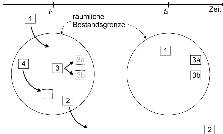
Abbildung 1: Skizze der vier allgemeinen Mechanismen der Bestandsdynamik bei Auszeichnung einer räumlichen Zugehörigkeitseigenschaft: Import (Element 1), Export (Element 2), Entstehen (Element 3) Vergehen (Element 4) von Elementen eines Bestandes. Die Kreise stellen die räumliche Grenze eines Bestandes an zwei verschiedenen Zeitpunkten dar, die Quadrate symbolisieren (hier der Übersichtlichkeit halber unterscheidbare) Elemente des Bestandes. Element 3 verdoppelt sich zwischen t_1 und t_2 zu zwei Elementen 3a und 3b, während Element 4 aufhört zu existieren.
