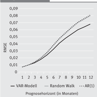
Vergleich RMSE
