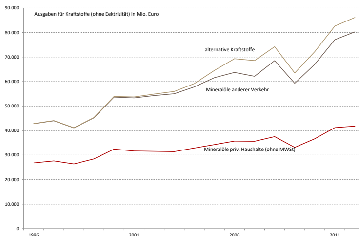
Abb. 7-6: Aggregierte Letztverbraucherausgaben für Verkehrsenergeträger
