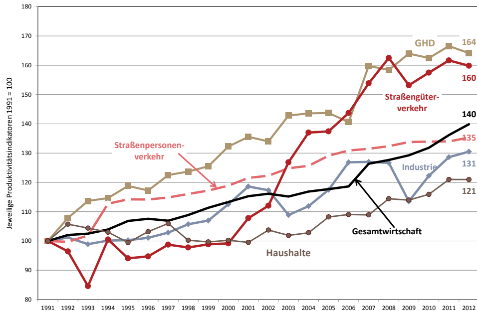
Abb. 3-7: Entwicklung der sektoralen Effizienzindikatoren in Deutschland von 1991 bis 2012
