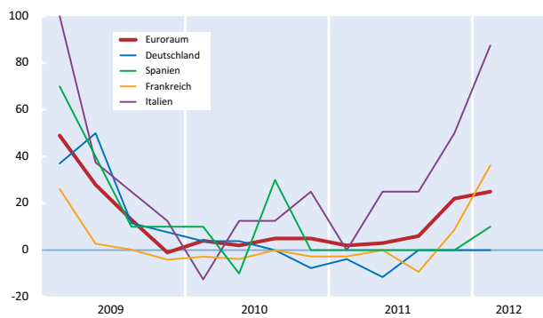
Abb. 5.4 Kreditrichtlinien a)
