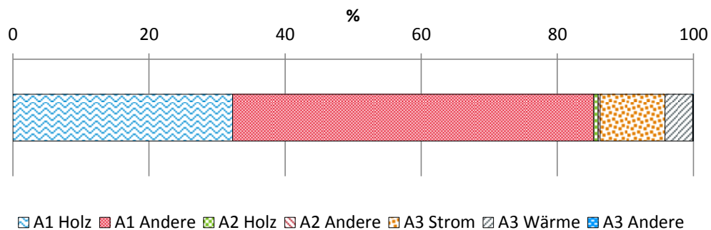
Abbildung 5.4.D: Relative Beiträge zum Parameter GWP (ohne holzinhärenten Kohlenstoff) für die Module A1 bis A3. Deklarierte Einheit ist 1 kg Küchenmöbel zzgl. Verpackung (Durchschnitt Küchenmöbel)
