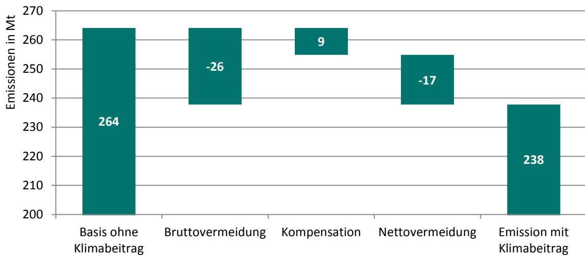
Abbildung 16: Brutto- und Nettovermeidung in 2020 durch Wechselwirkung mit den Nachbarländern
