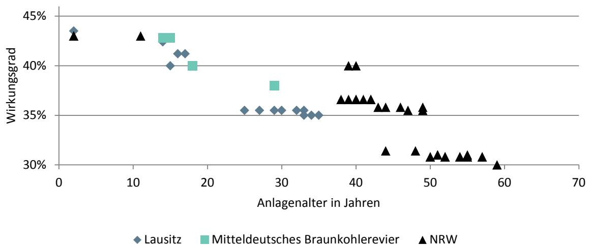
Abbildung 6: Regionale Verteilung, Alter und Wirkungsgrade der Braunkohlekraftwerke Quelle: Eigene Darstellung basierend auf BNetzA (2014b) und eigenen Annahmen.
