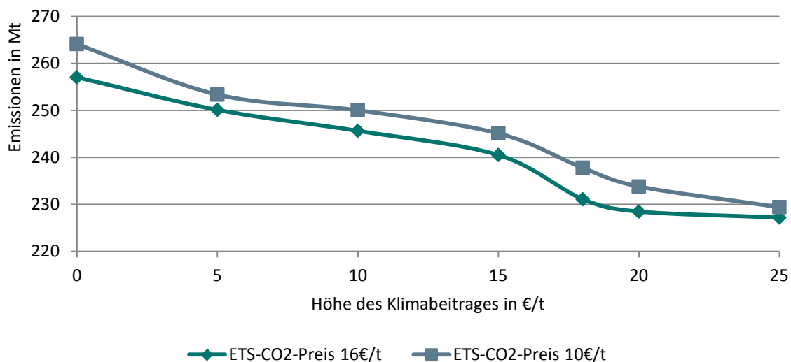
Abbildung 24: Emissionen in Deutschland je nach CO 2 -Preis und Höhe des Klimabeitrags
