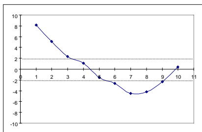
2.e). Spatial distribution, monocentre (case 3.2)
