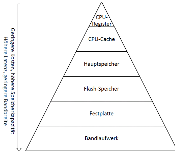
Abbildung 3.1.: Die Speicherhierarchie.
