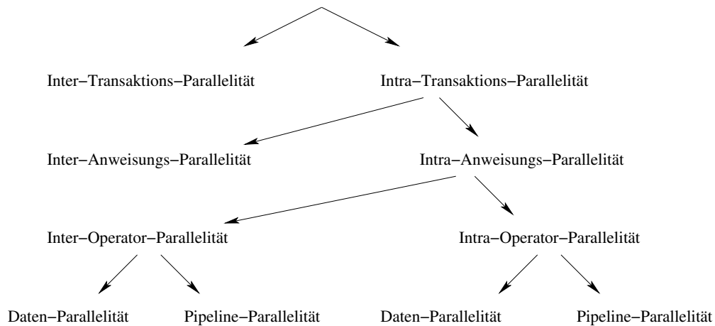
Abbildung 3.3.: Arten von Parallelverarbeitung.
