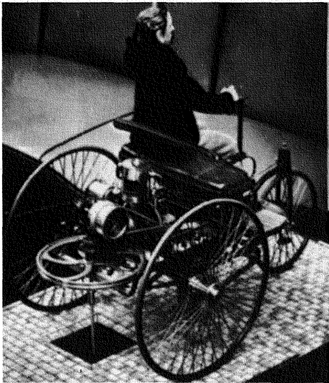
Der erste Motorwagen von Carl Benz aus dem Jahre 1885.
