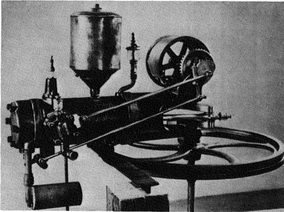
Motor des ersten dreirädrigen Motorwagens von Carl Benz aus dem Jahre 1885.
