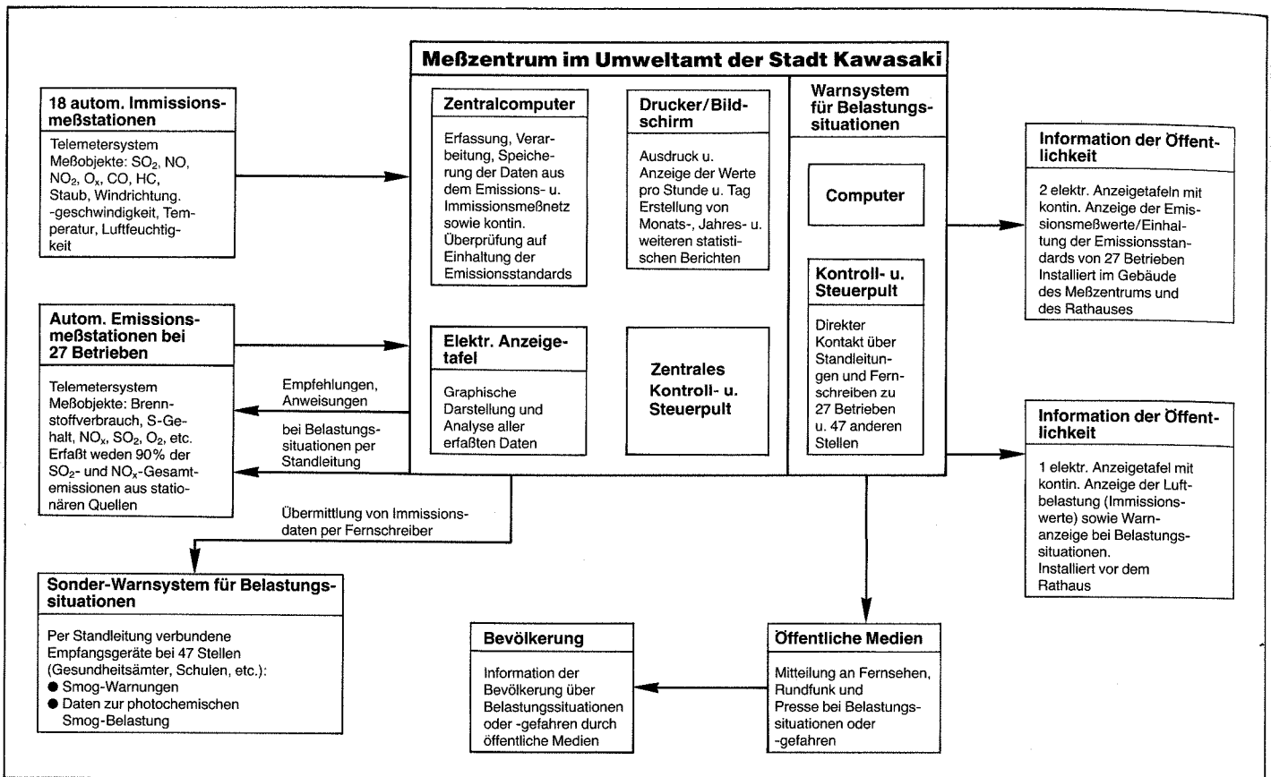
Abb. 1: Überwachungs- und Warnsystem (Immissionsschutz) in Kawasaki
