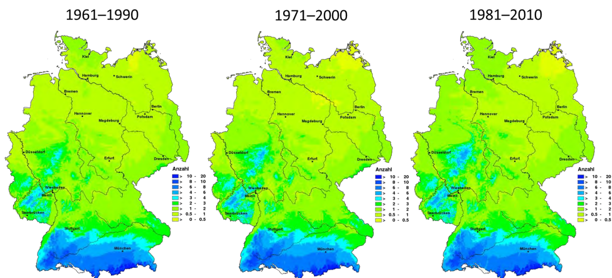
Abbildung 2.29: Häufigkeit des Auftretens einer Niederschlagssumme von mehr als 50 mm innerhalb von 3 Tagen im Jahr, 30-jährigen Mittelwerte 1961-1990, 1971-2000, 2000, 1981-2010
