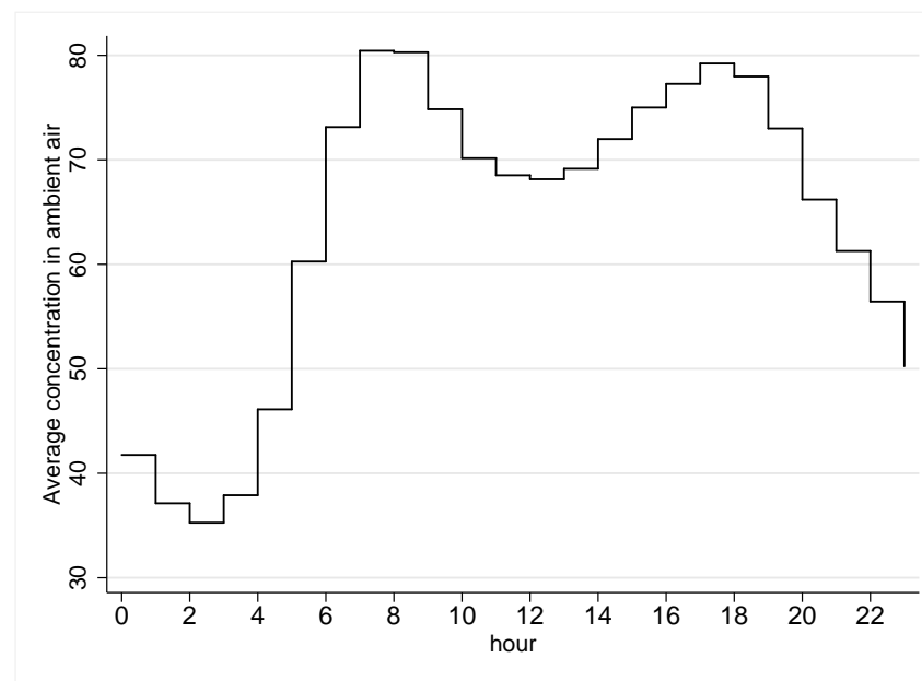
(b) NO2
