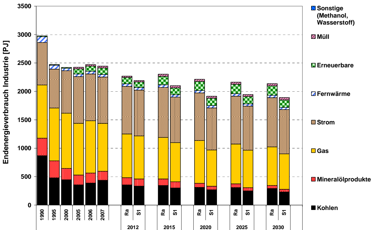
Abbildung 11.3: Endenergieverbrauch im Industriesektor in der Sensitivitätsanalyse „Die Krise dauert länger“ (S1) im Vergleich zur Referenzprognose (Ra)
