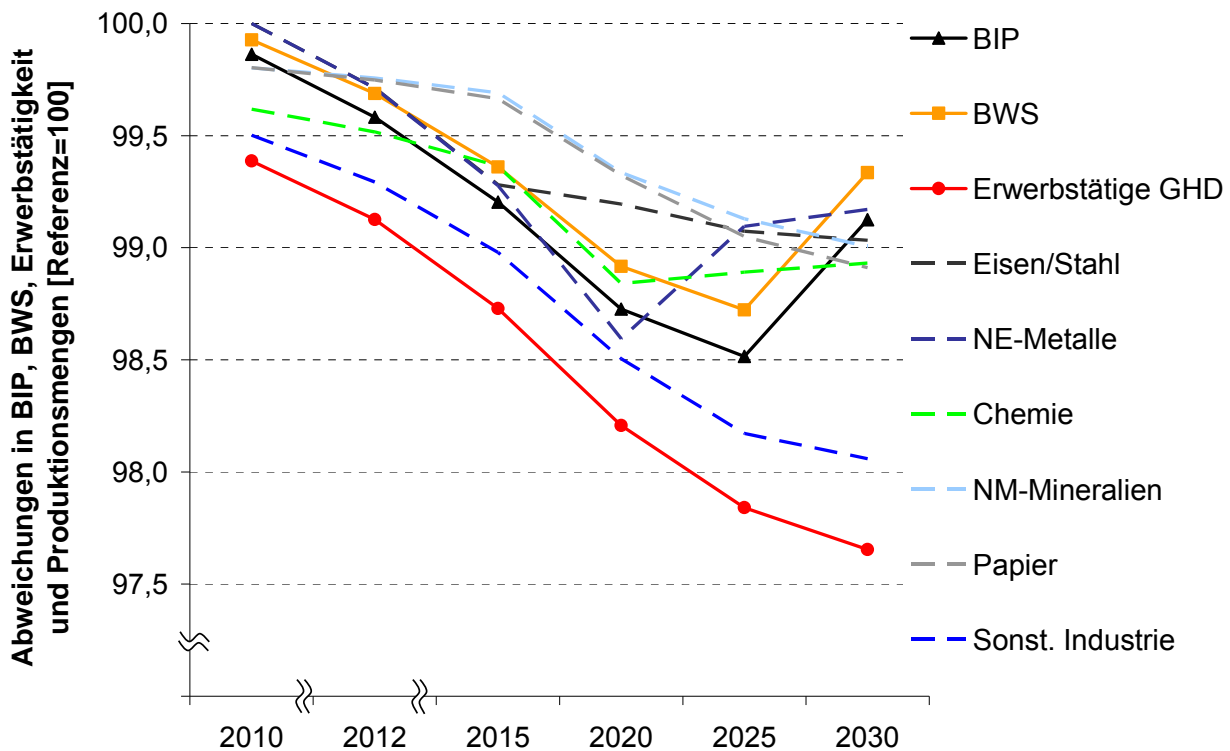
Abbildung 11.4: Veränderungen prognoserelevanter Inputgrößen in der Sensitivitätsanalyse „Hohe Ölpreise bei Kernenergieausstieg“ (S2a) gegenüber der Referenzprognose (Ra)
