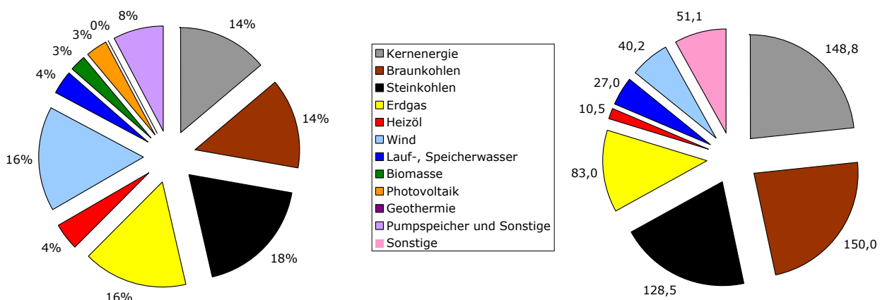
Abbildung 3.14: Anteil an der installierten elektrischen Netto-Engpassleistung (links, insgesamt 147,089 GW) und bereitgestellte elektrische Arbeit (rechts, brutto in TWh) in 2008 nach Energieträgern, BDEW (2009a)
