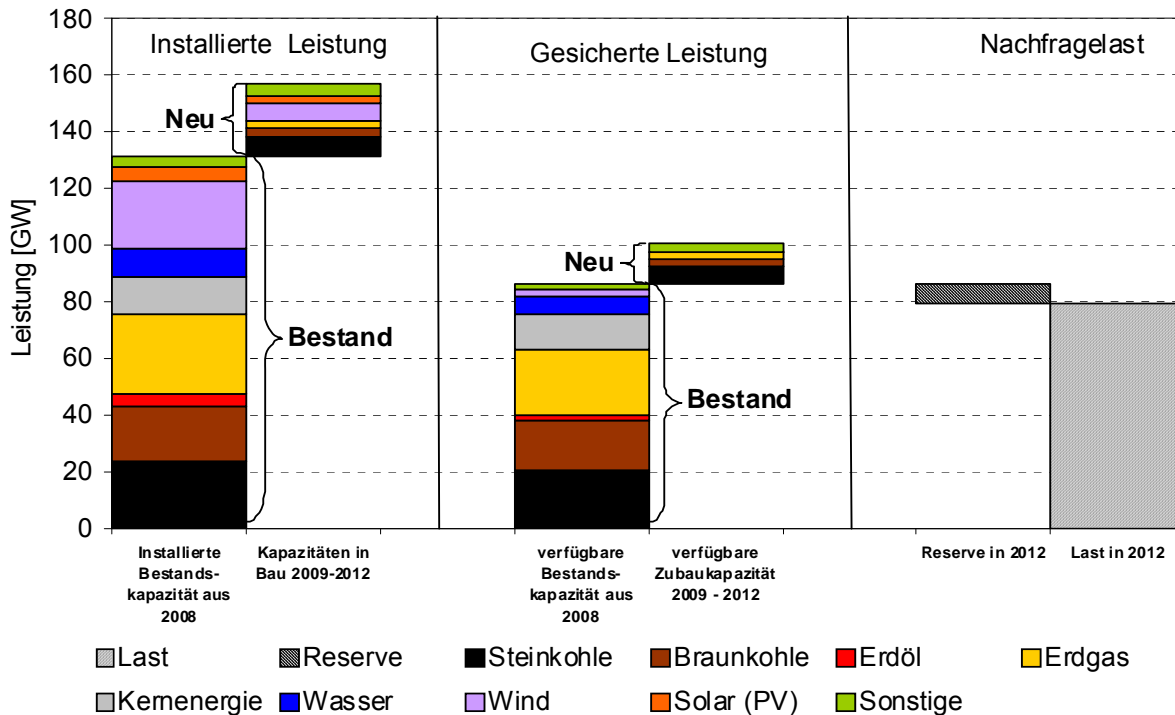
Abbildung 4.17: Kraftwerkskapazitäten und Nachfragelast zur Spitzenlastzeit in Deutschland in 2012 in der Referenzprognose (Ra)
