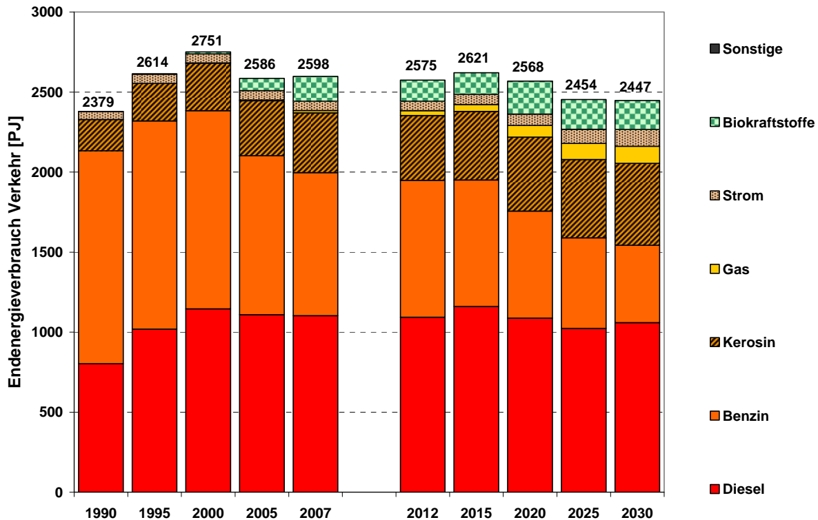
Abbildung 5.8: Endenergieverbrauch des Verkehrssektors in der Variante mit Laufzeitverlängerung (Rb)
