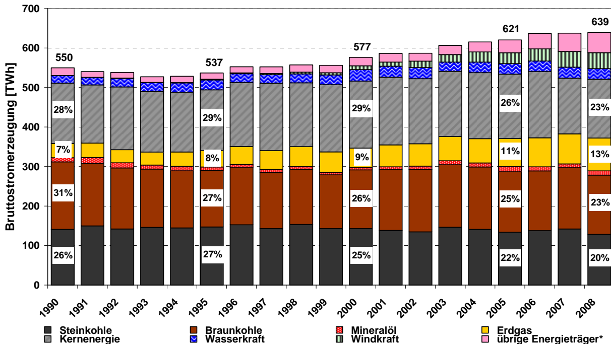
Abbildung 10.4: Bruttostromerzeugung nach Energieträgern in Deutschland
