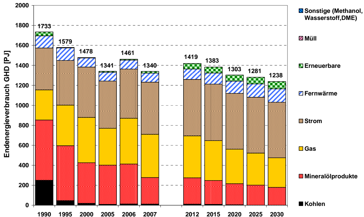
Abbildung 4.7: Entwicklung des Endenergieverbrauchs des Sektors Gewerbe, Handel, Dienstleistungen (GHD) in der Referenzprognose (Ra)
