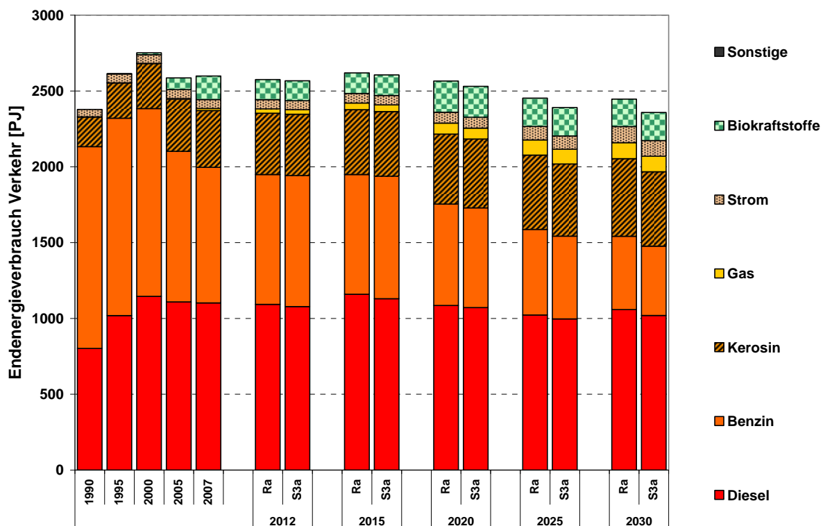
Abbildung 11.11: Endenergieverbrauch im Verkehrssektor in der Sensitivitätsanalyse „Verstärkter Klimaschutz bei Kernenergieausstieg“ (S3a) im Vergleich zur Referenzprognose (Ra)
