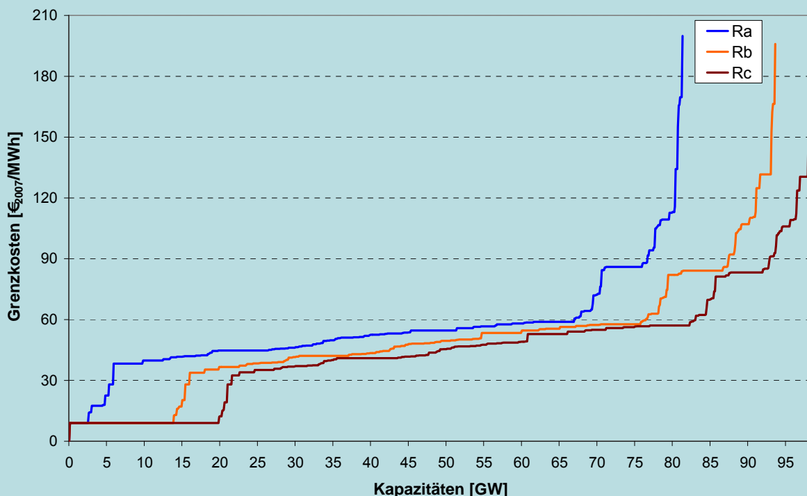
Abbildung 5.22: Merit-Order-Kurve der thermischen Erzeugungskapazitäten in Deutschland an einem repräsentativen Wintertag in 2020 für die Variante „Laufzeitverlängerung der Kernkraftwerke auf 60 Jahre“ (Rc) im Vergleich zur Referenzprognose (Ra) und zur Variante mit Laufzeitverlängerung auf 40 Jahre (Rb)
