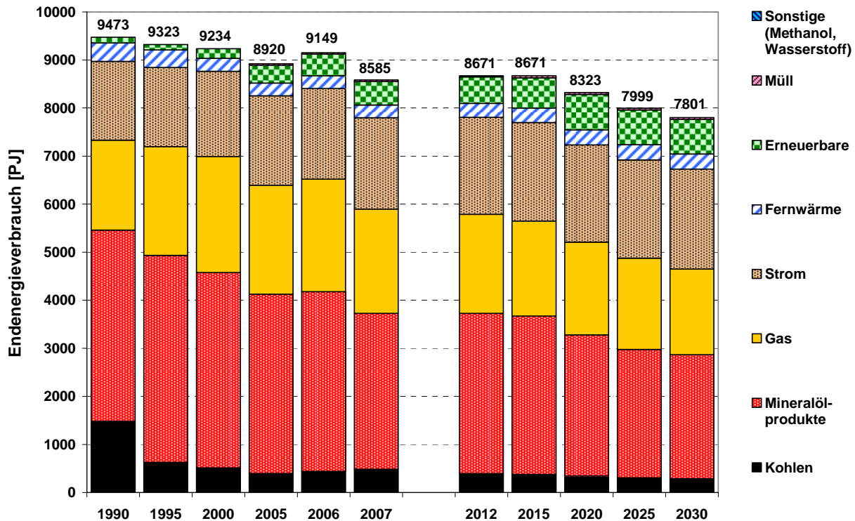
Abbildung 5.9: Endenergieverbrauch nach Energieträgern in der Variante mit Laufzeitverlängerung (Rb)
