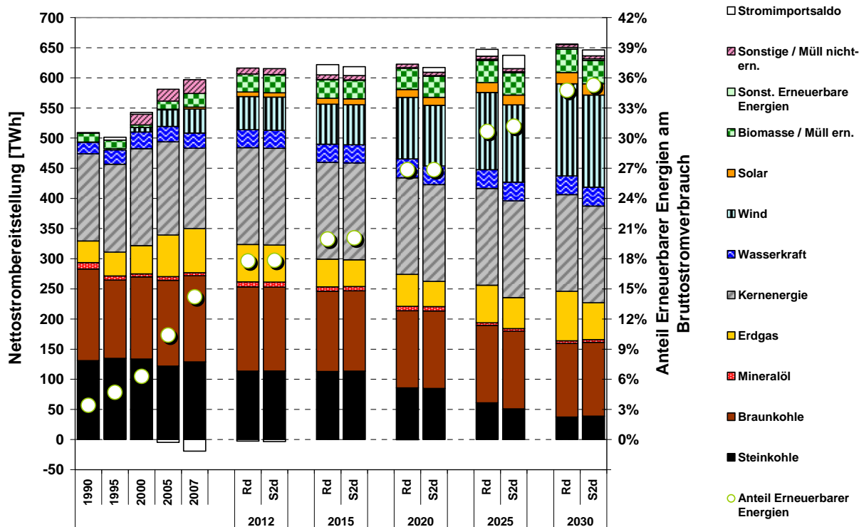
Abbildung 11.9: Nettostrombereitstellung in der Sensitivitätsanalyse „Hohe Ölpreise bei Laufzeitverlängerung“ (S2d) im Vergleich zur Variante mit Laufzeitverlängerung (Rd)
