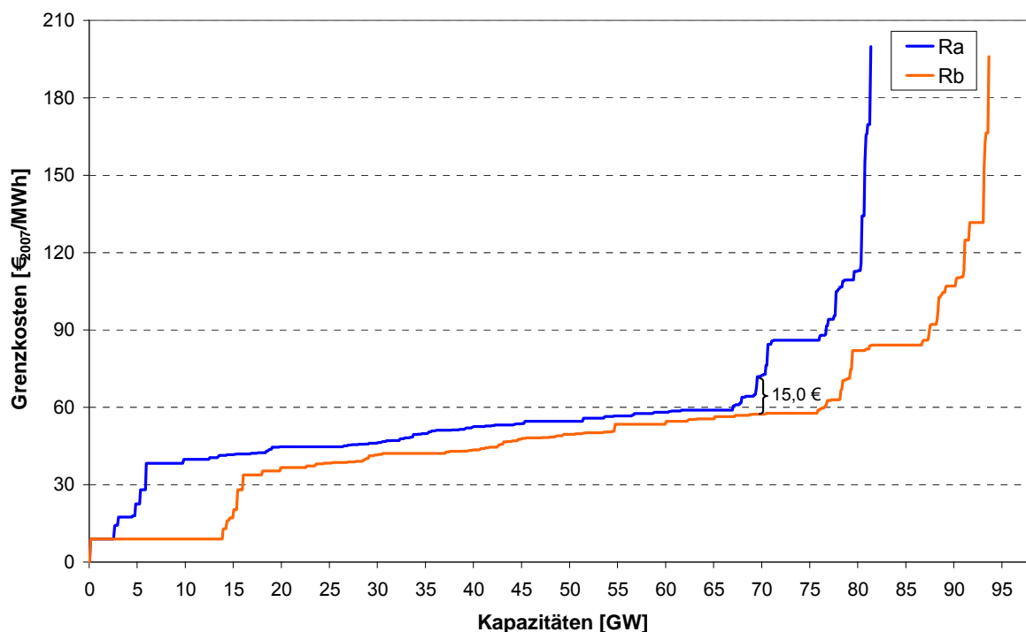
Abbildung 5.1: Merit-Order-Kurven der thermischen Erzeugungskapazitäten in Deutschland an einem repräsentativen Wintertag in 2020 für die Referenzprognose (Ra) und für die Variante mit Laufzeitverlängerung (Rb)
