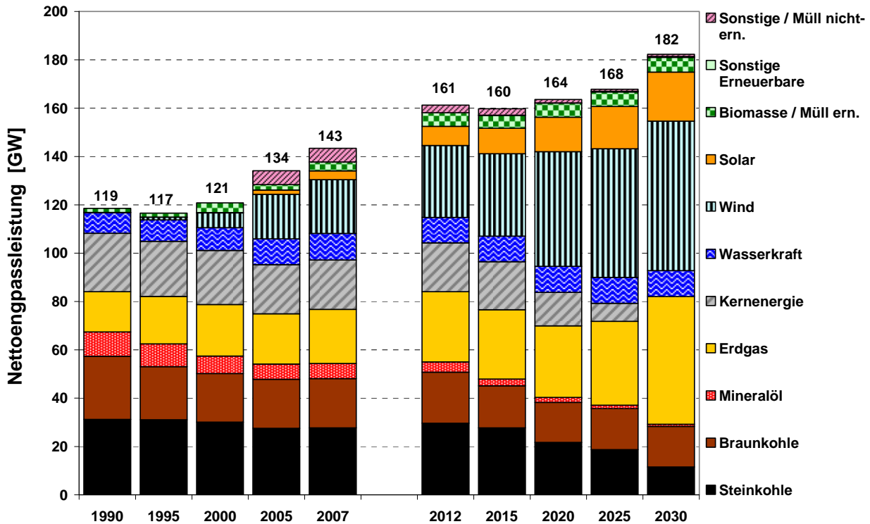
Abbildung 5.13: Nettoengpassleistung in Deutschland in der Variante mit Laufzeitverlängerung (Rb)
