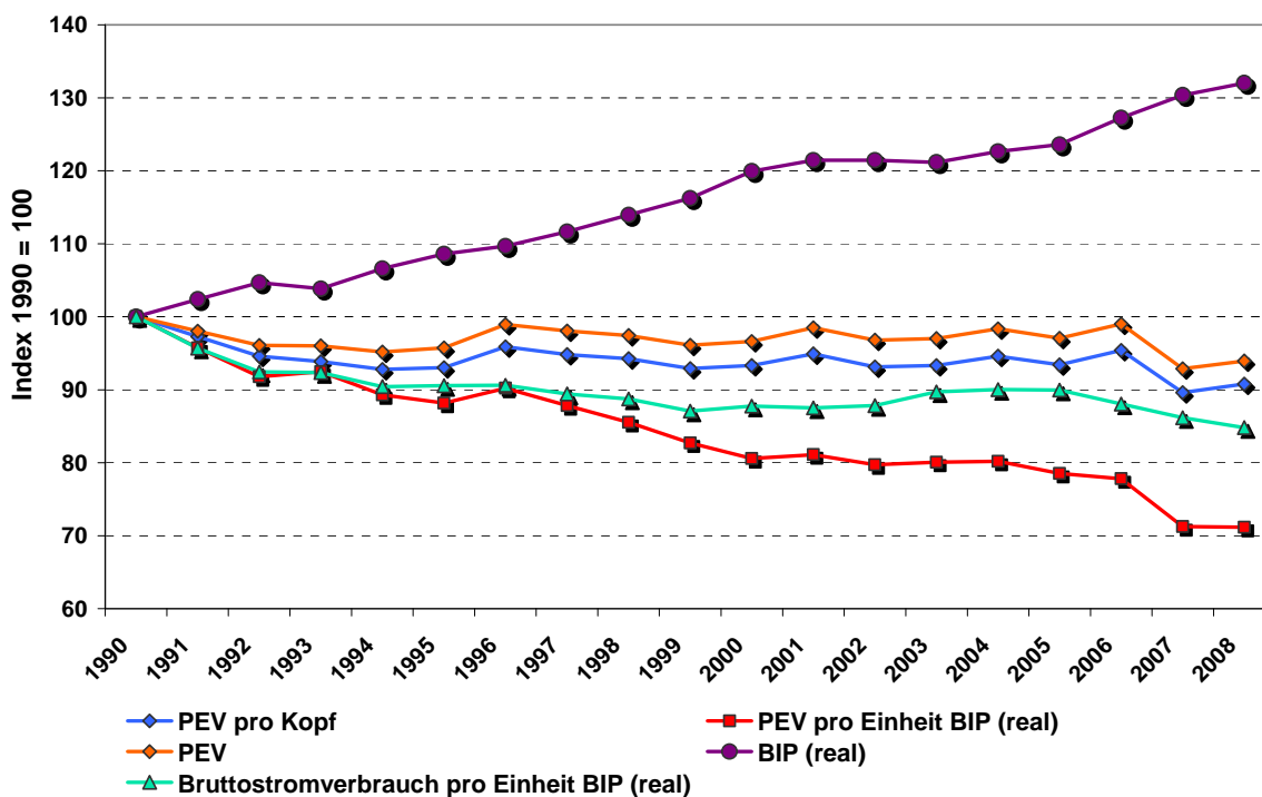
Abbildung 10.7: Wesentliche Energieindikatoren für Deutschland im Überblick
