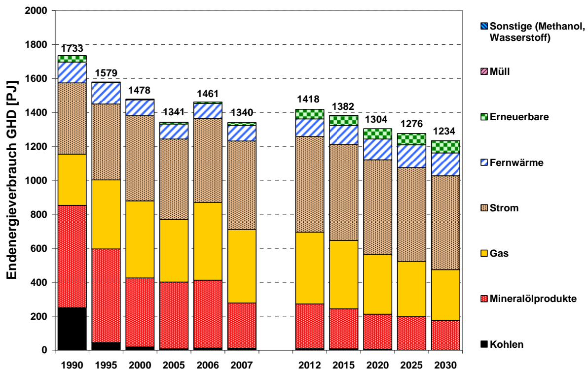
Abbildung 5.6: Entwicklung des Endenergieverbrauchs des Sektors Gewerbe, Handel, Dienstleistungen (GHD) in der Variante mit Laufzeitverlängerung (Rb)
