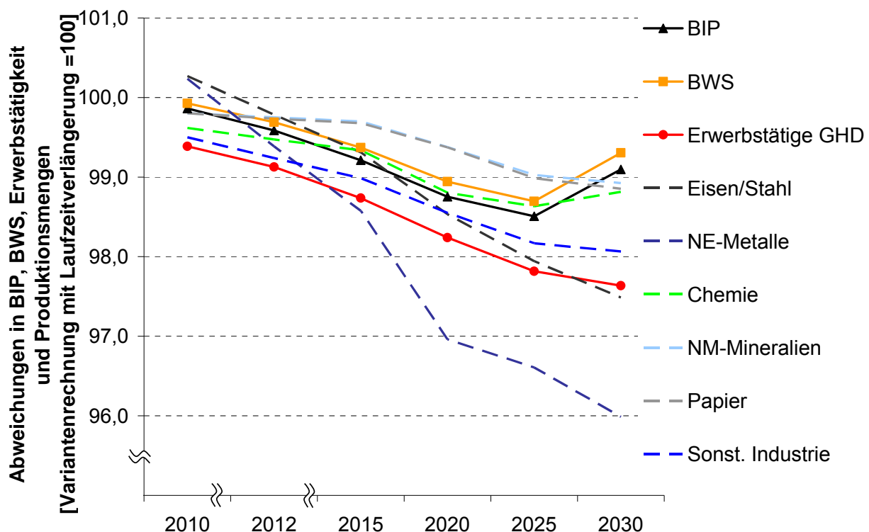
Abbildung 11.7: Veränderungen prognoserelevanter Inputgrößen in der Sensitivitätsanalyse „Hohe Ölpreise bei Laufzeitverlängerung“ (S2d) gegenüber der Variante mit Laufzeitverlängerung (Rd)
