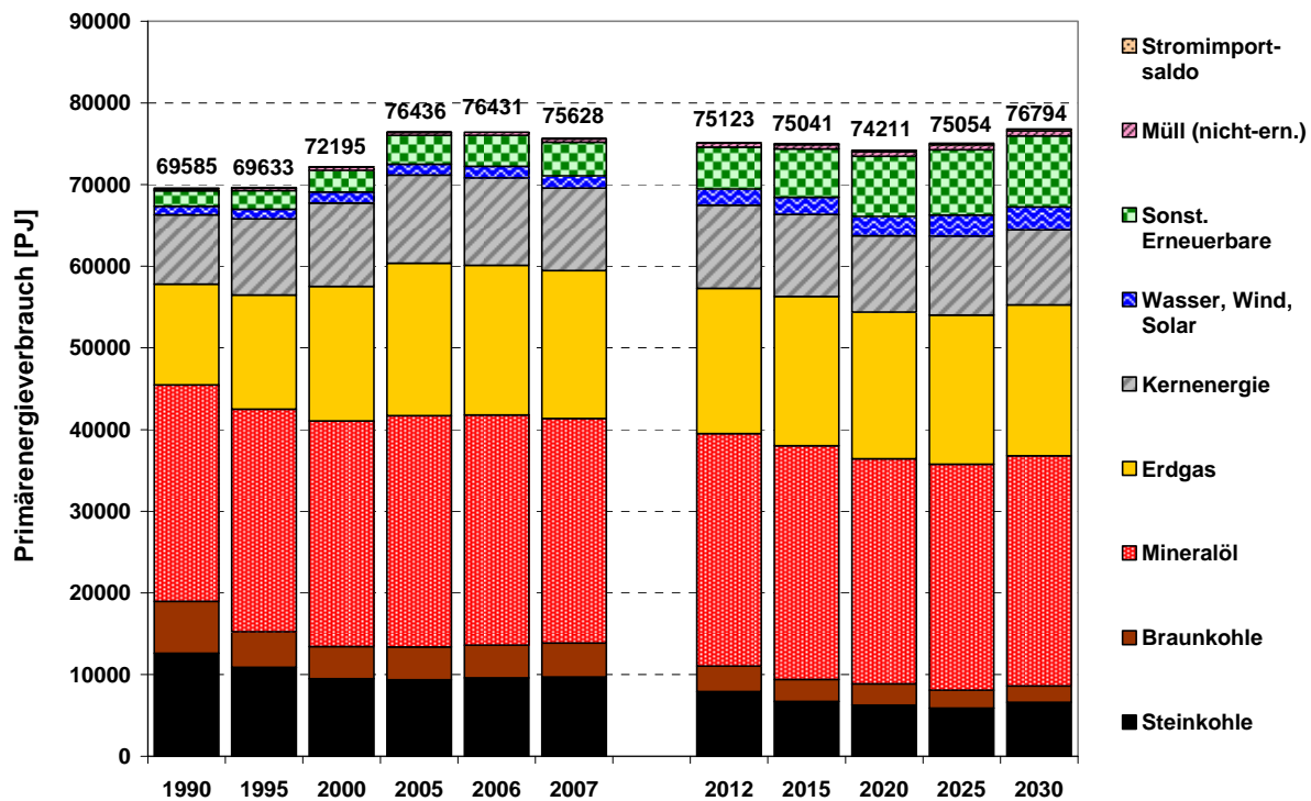
Abbildung 4.1: Primärenergieverbrauch in der EU-27 nach Energieträgern in der Referenzprognose (Ra)
