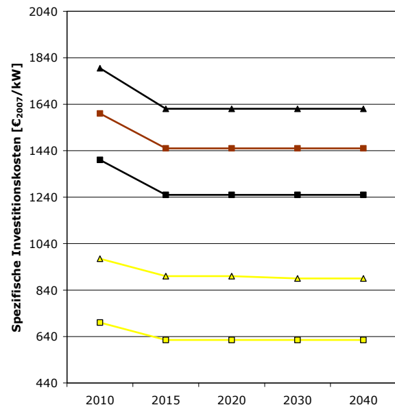
Abbildung 3.16: Entwicklung von Wirkungsgraden und Investitionskosten ausgewählter konventioneller Wärmekraftwerke
