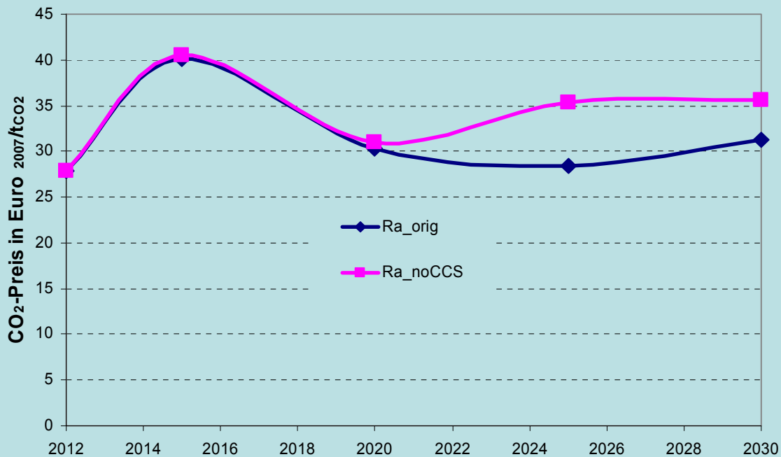
Abbildung 4.23: CO 2 -Preis in der Referenzprognose (Ra) und in der Sensitivitätsanalyse „CCS wird nicht marktfähig“ (Ra_NoCCS)
