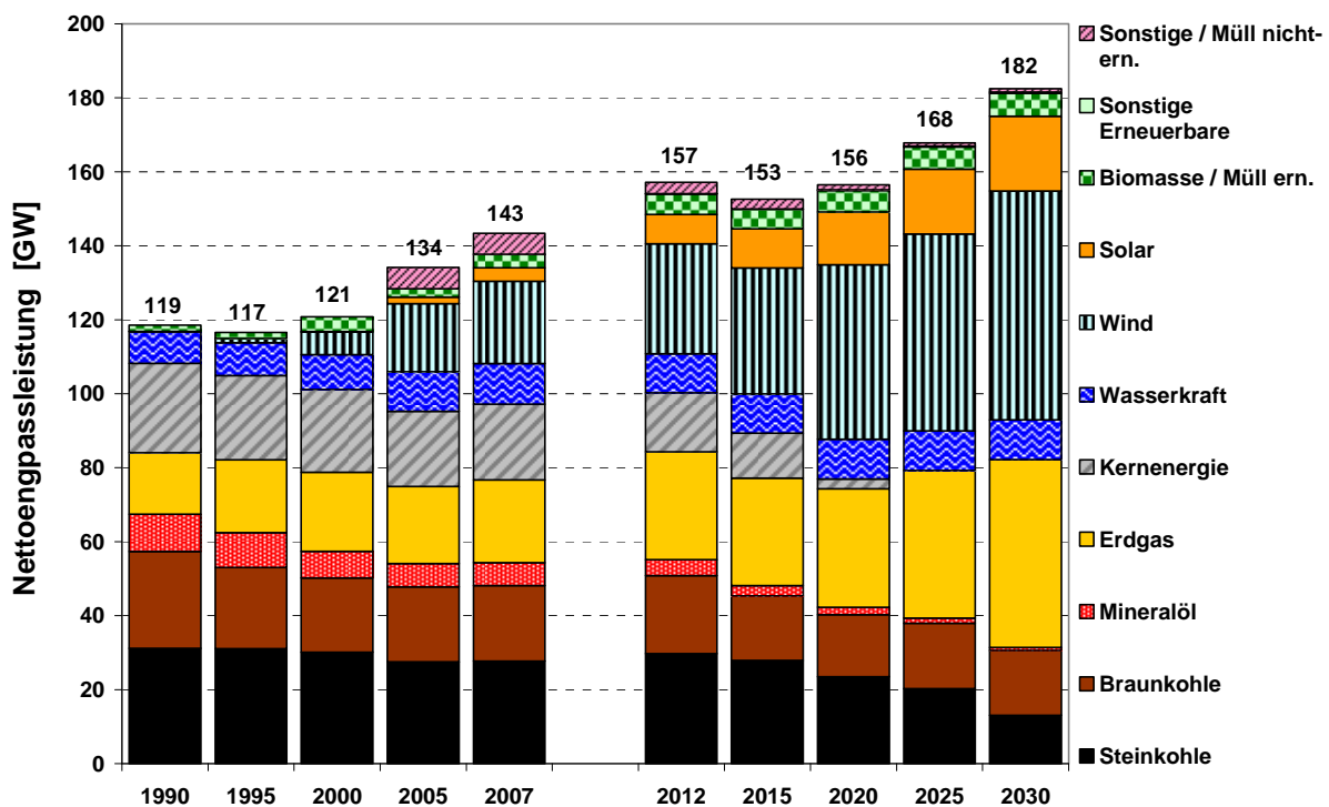
Abbildung 4.16: Nettoengpassleistung in Deutschland in der Referenzprognose (Ra)
