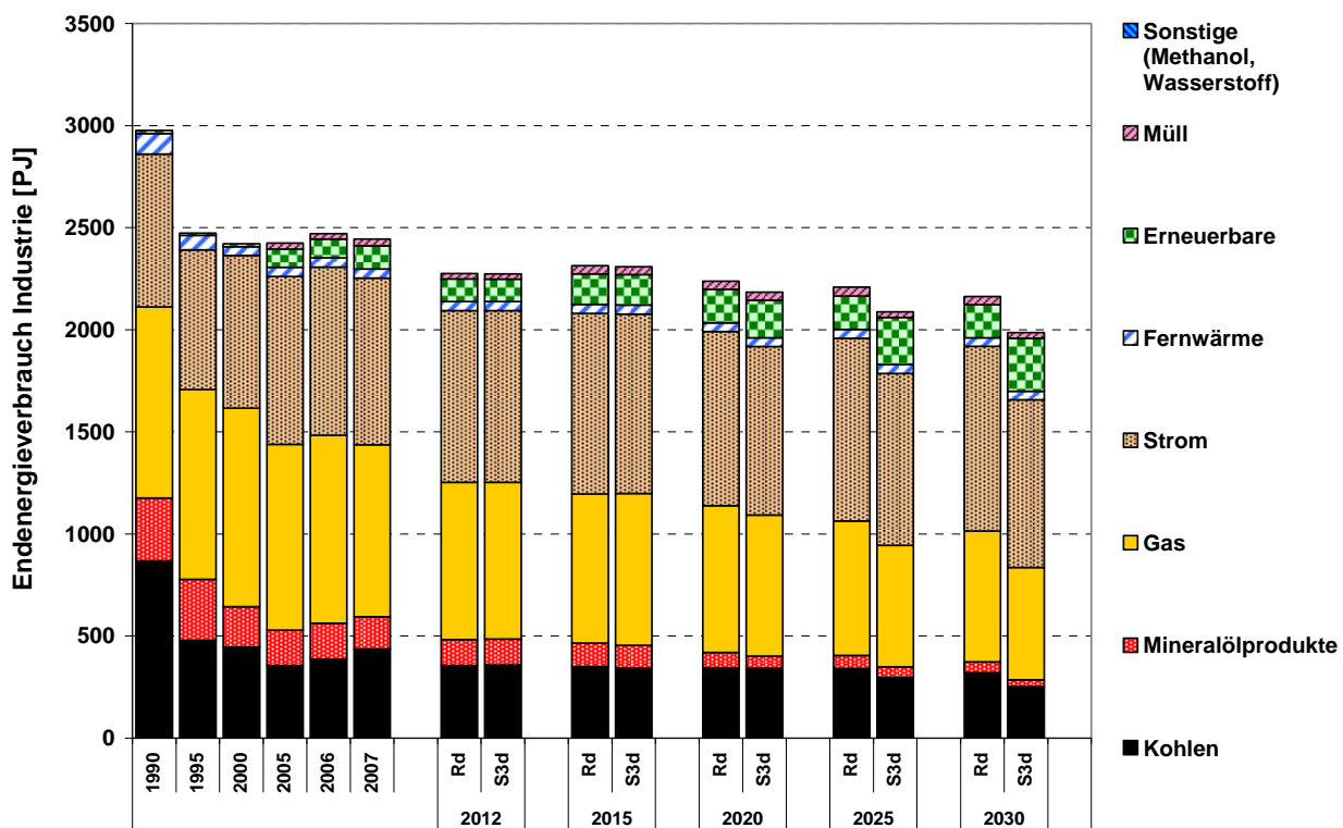
Abbildung 11.14: Endenergieverbrauch der Industrie in der Sensitivitätsanalyse „Verstärkter Klimaschutz bei Laufzeitverlängerung“ (S3d) im Vergleich zur Variante mit Laufzeitverlängerung (Rd)
