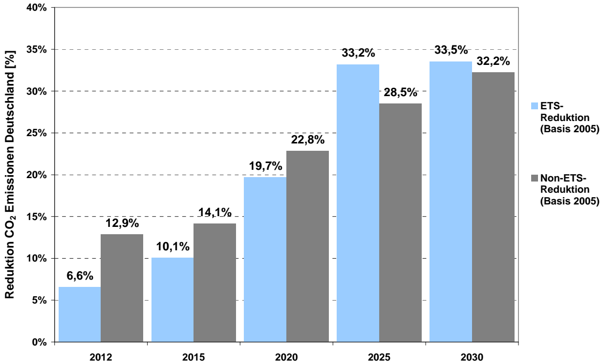
Abbildung 4.30: Reduktion der CO 2 -Emissionen in Deutschland im ETS- bzw. Nicht-ETS-Sektor in der Referenzprognose (Ra)
