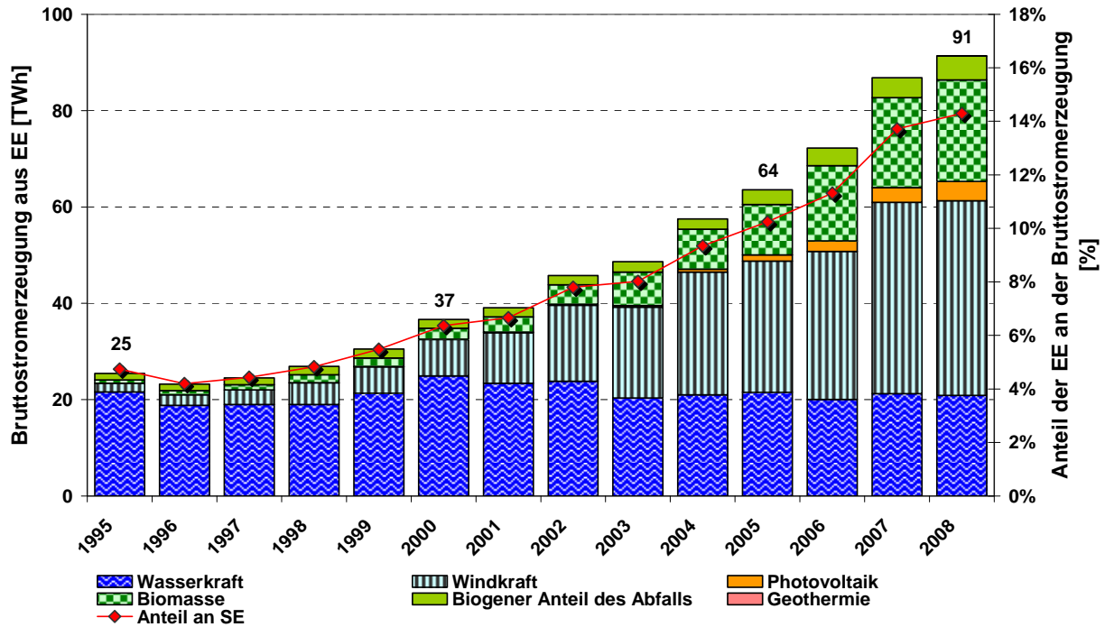
Abbildung 10.5: Beitrag der Erneuerbaren Energien zur Bruttostromerzeugung in Deutschland
