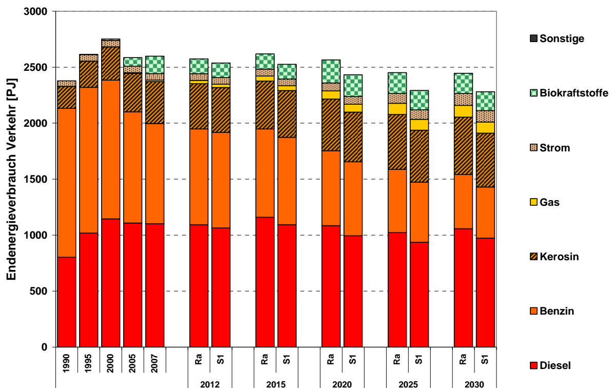
Abbildung 11.2: Endenergieverbrauch im Verkehrssektor in der Sensitivitätsanalyse „Die Krise dauert länger“ (S1) im Vergleich zur Referenzprognose (Ra)
