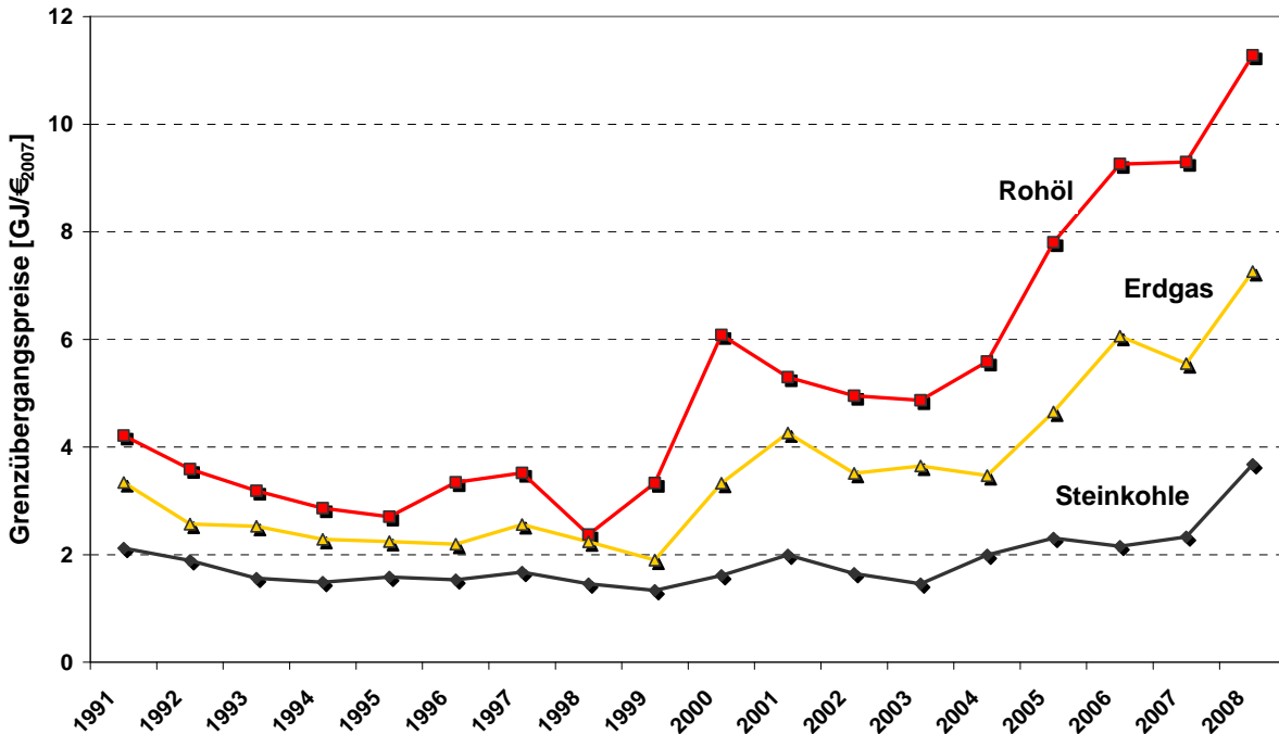
Abbildung 10.1: Reale Grenzübergangspreise wichtiger fossiler Energieträger (Jahresdurchschnittswerte)
