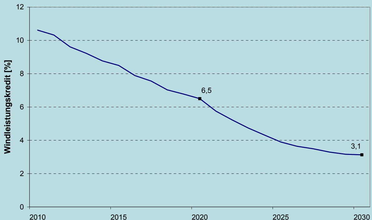
Abbildung 4.19: Leistungskredit der Windkonverter in der Referenzprognose (Ra)
