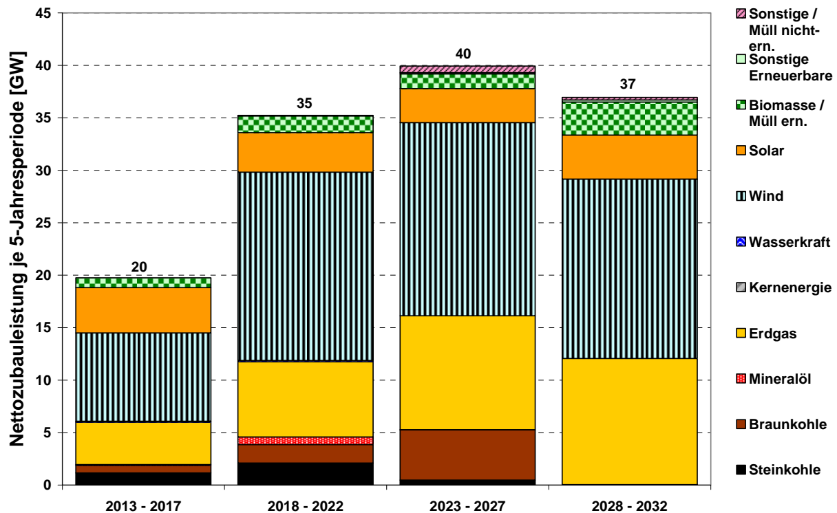
Abbildung 4.18: Zubaukapazitäten in Deutschland nach 2012 in der Referenzprognose (Ra)
