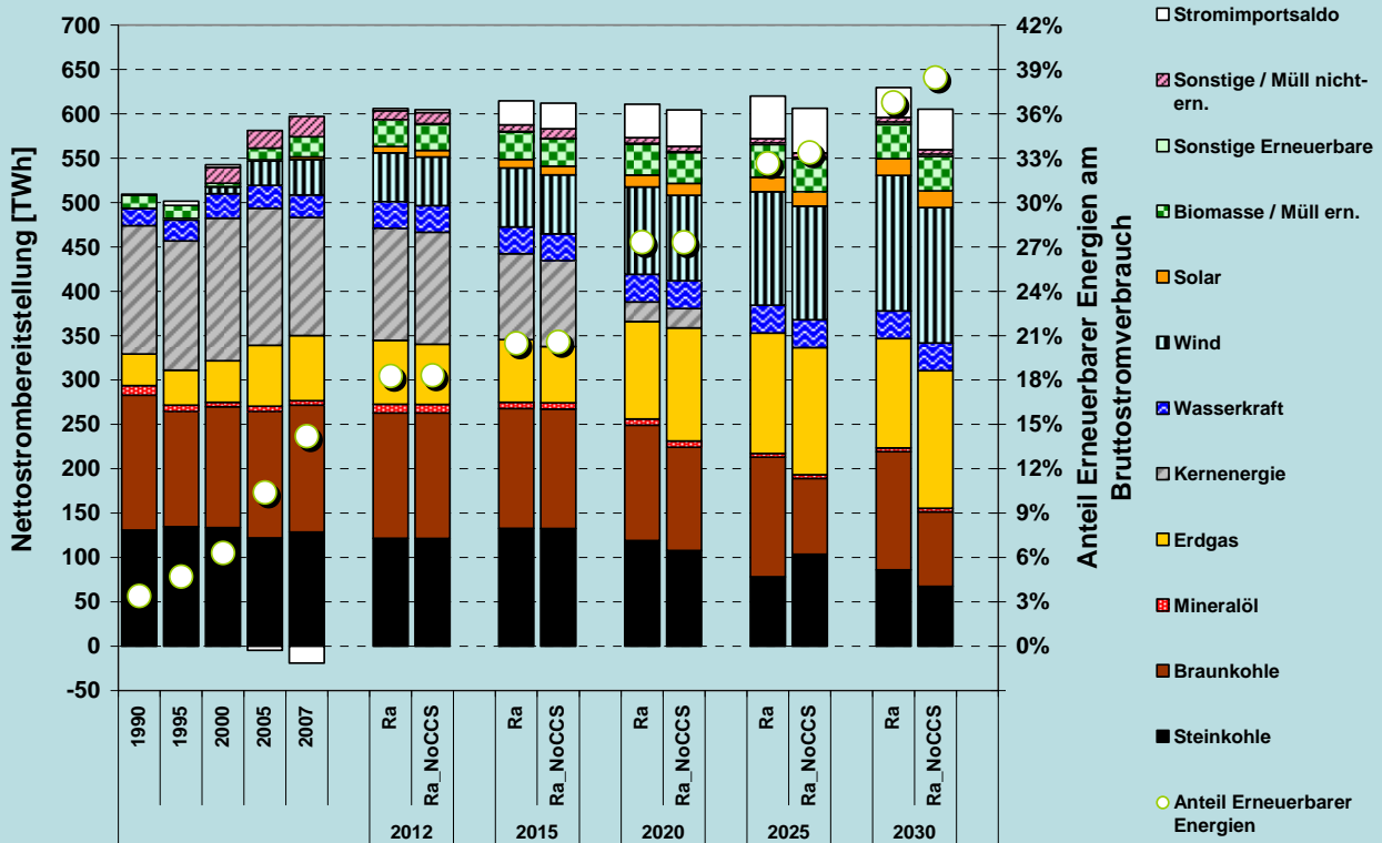
Abbildung 4.25: Nettostrombereitstellung in der Referenzprognose (Ra) und in der Sensitivitätsanalyse „CCS wird nicht marktfähig“ (Ra_NoCCS)
