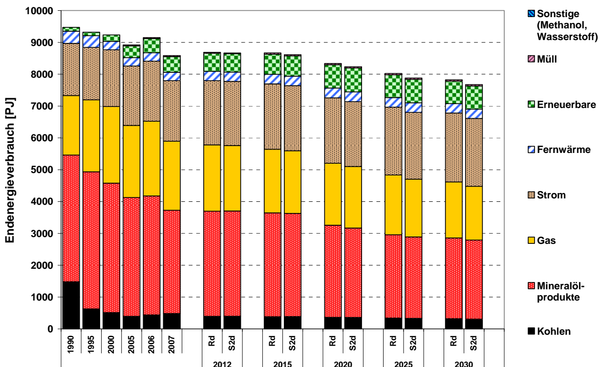
Abbildung 11.8: Endenergieverbrauch in der Sensitivität „Hohe Ölpreise bei Laufzeitverlängerung“ (S2d) im Vergleich zur Variante mit Laufzeitverlängerung (Rd)
