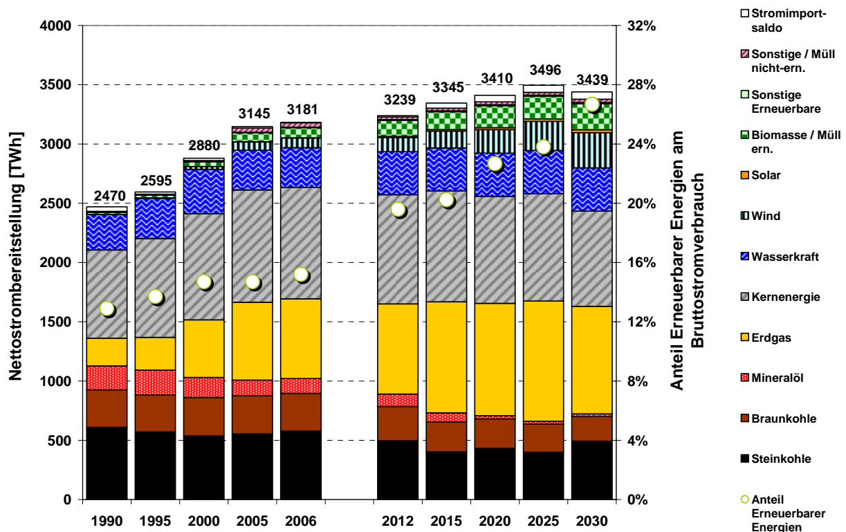
Abbildung 5.12: Nettostrombereitstellung in der EU-27 in der Variante mit Laufzeitverlängerung (Rb)
