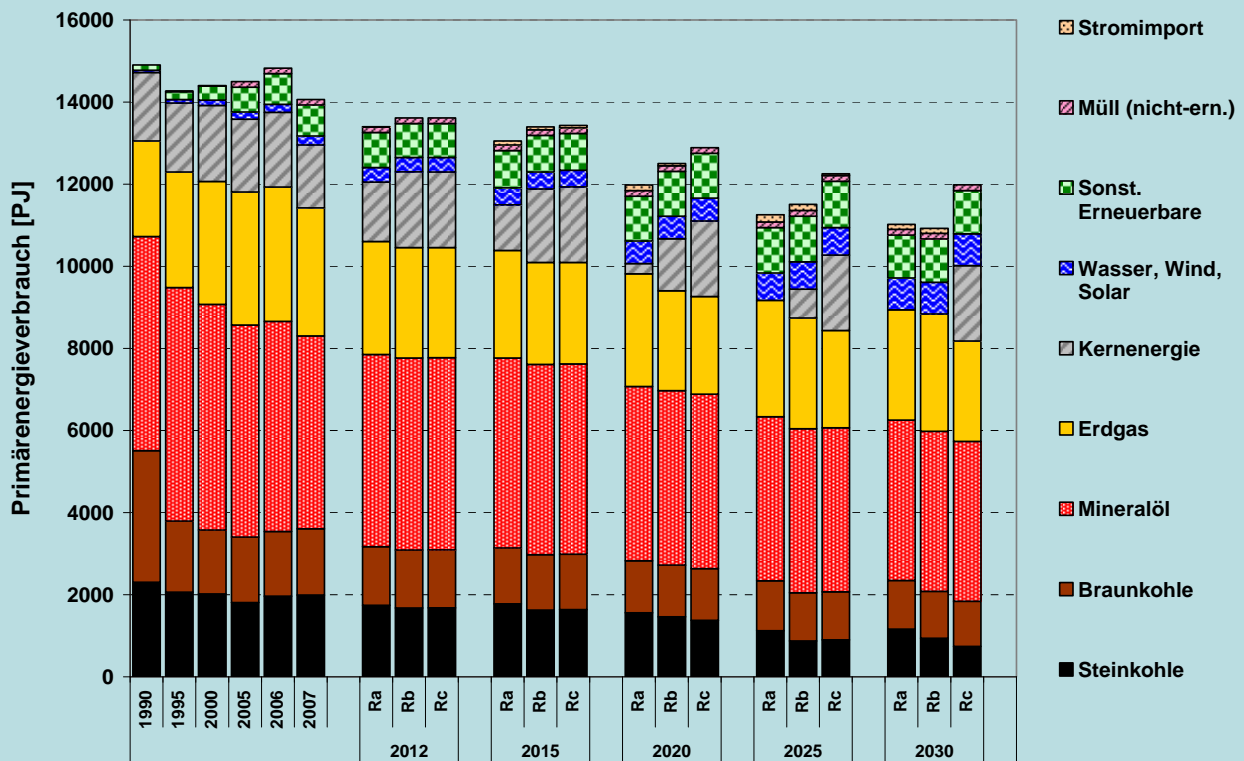
Abbildung 5.23: Primärenergieverbrauch in der Variante Laufzeitverlängerung der Kernkraftwerke auf 40 Jahre (Rc) im Vergleich zur Referenzprognose (Ra) und zur Variante mit Laufzeitverlängerung auf 60 Jahre (Rb)
