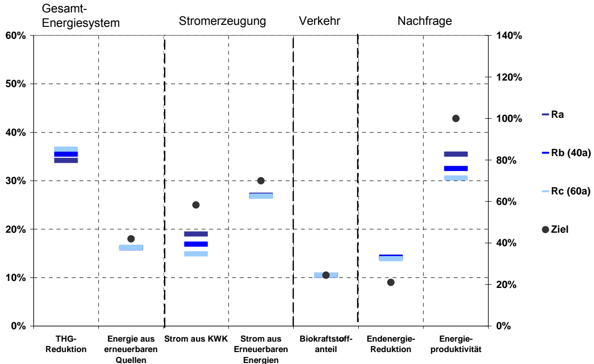
Abbildung 5.24: Vergleich energie- und klimapolitischer Ziele mit den Entwicklungen in der Referenzprognose bei Kernenergieausstieg (Ra) und in den Varianten mit Laufzeitverlängerung (Rb, Rc)
