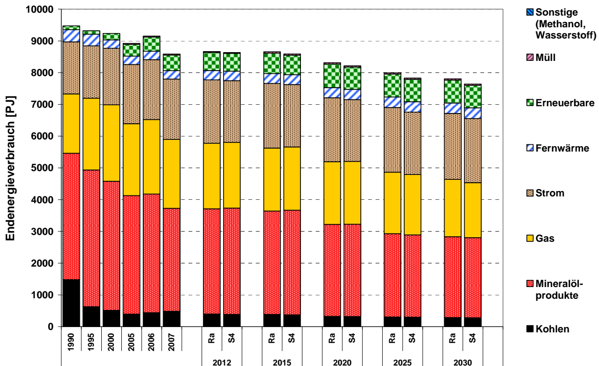
Abbildung 11.17: Endenergieverbrauch in der Sensitivitätsanalyse „Niedrigere Bevölkerungsentwicklung“ (S4) im Vergleich zur Referenzprognose (Ra)
