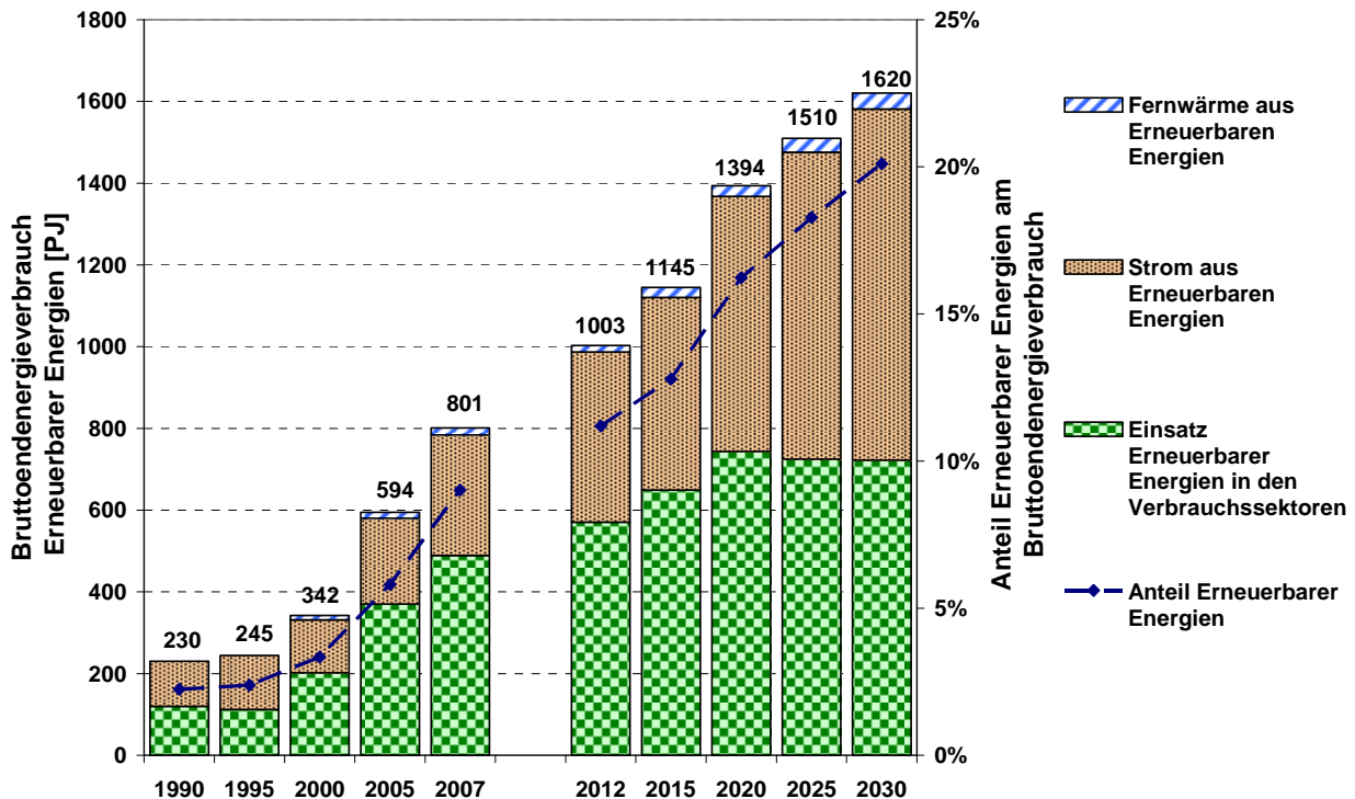
Abbildung 4.28: Anteil der Erneuerbaren Energien am Bruttoendenergieverbrauch in der Referenzprognose (Ra)
