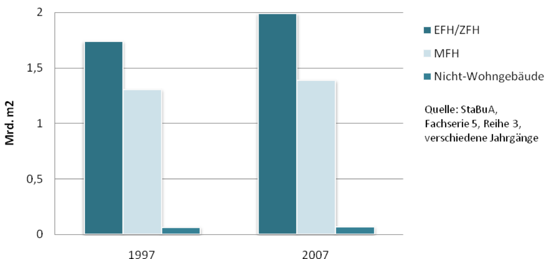
Abbildung 3.6: Wohnflächenbestand 1997 und 2007
