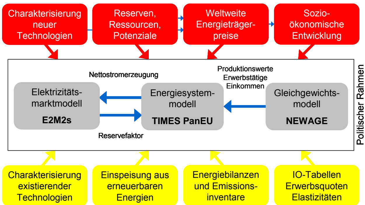
Abbildung 1.1: Modellinstrumentarium
