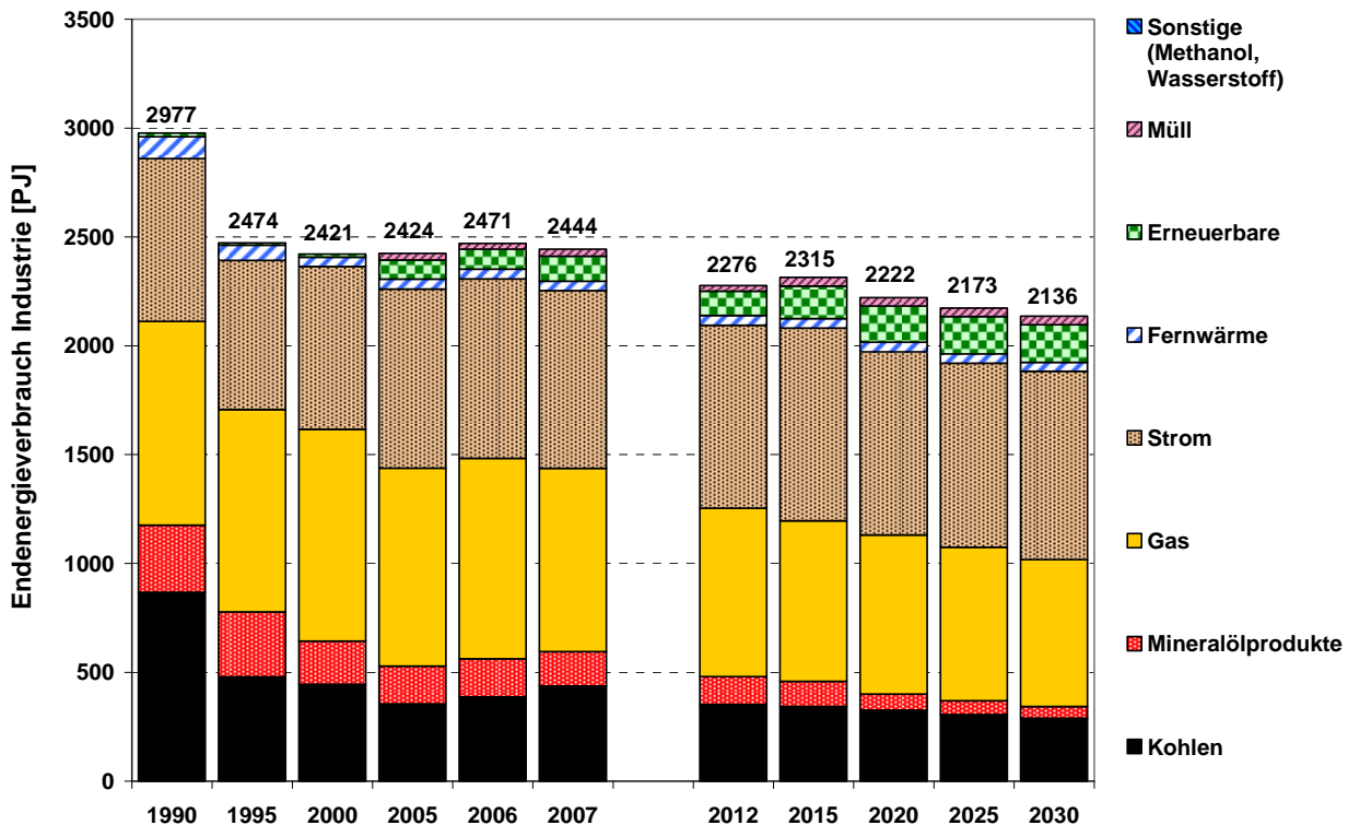
Abbildung 5.5: Endenergieverbrauch der Industrie in der Variante mit Laufzeitverlängerung (Rb)
