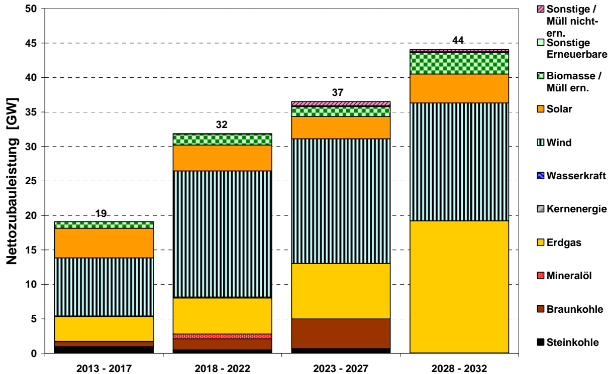
Abbildung 5.14: Zubaukapazitäten in Deutschland nach 2012 in der Variante mit Laufzeitverlängerung (Rb)
