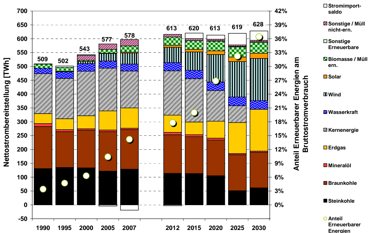
Abbildung 5.11: Nettostrombereitstellung in Deutschland in der Variante mit Laufzeitverlängerung (Rb)
