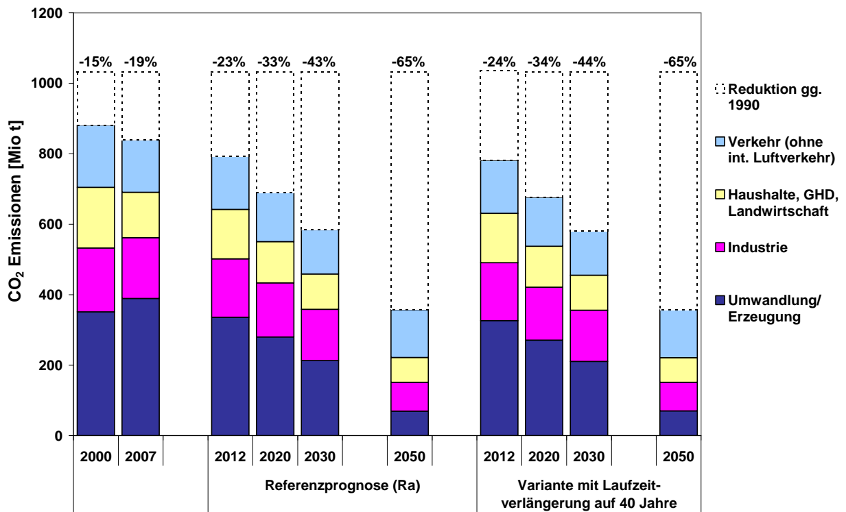
Abbildung 8.4: Ausblick 2050 zur Entwicklung der CO 2 -Emissionen in Deutschland in der Referenzprognose (Ra) (links) und in der Variante mit Laufzeitverlängerung (Rb) (rechts)
