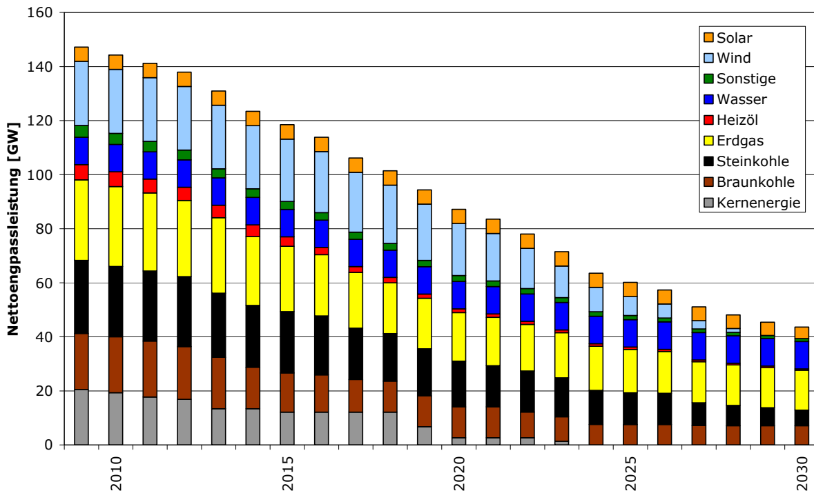
Abbildung 3.15: Kraftwerkssterbelinie des Anfang 2009 in Deutschland bestehenden Kraftwerks-parks bei Kernenergieausstieg
