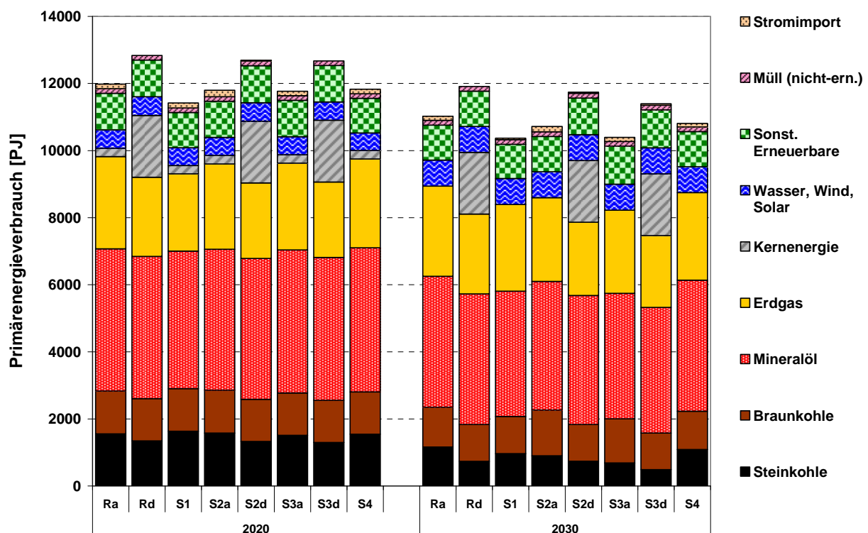
Abbildung 6.1: Primärenergieverbrauch der Jahre 2020 und 2030 in den Sensitivitätsanalysen
