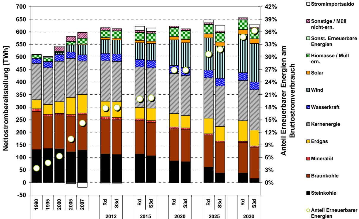
Abbildung 11.15: Nettostrombereitstellung in der Sensitivitätsanalyse „Verstärkter Klimaschutz bei Laufzeitverlängerung“ (S3d) im Vergleich zur Variante mit Laufzeitverlängerung (Rd)
