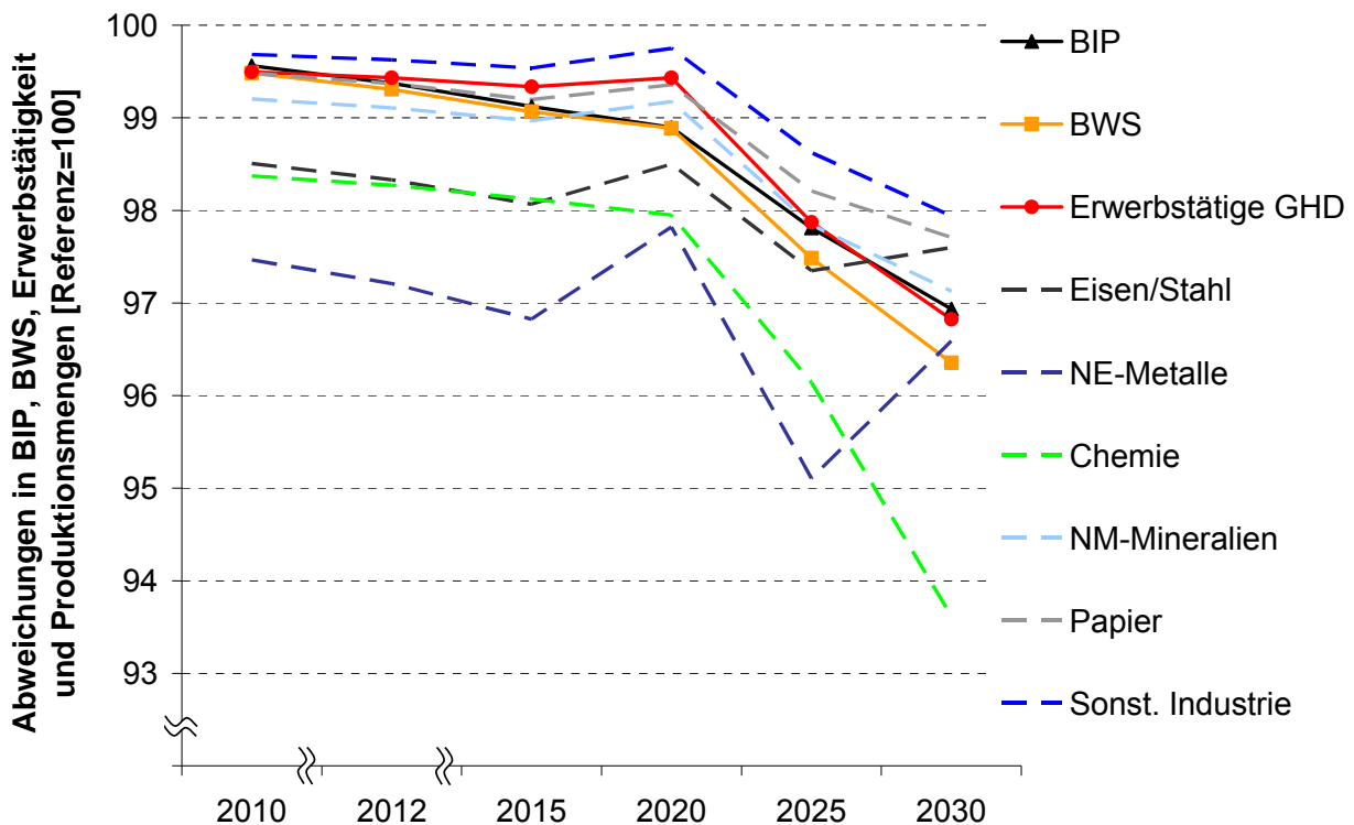
Abbildung 11.10: Veränderungen prognoserelevanter Inputgrößen in der Sensitivitätsanalyse „Verstärkter Klimaschutz bei Kernenergieausstieg“ (S3a) gegenüber der Referenzprognose (Ra)
