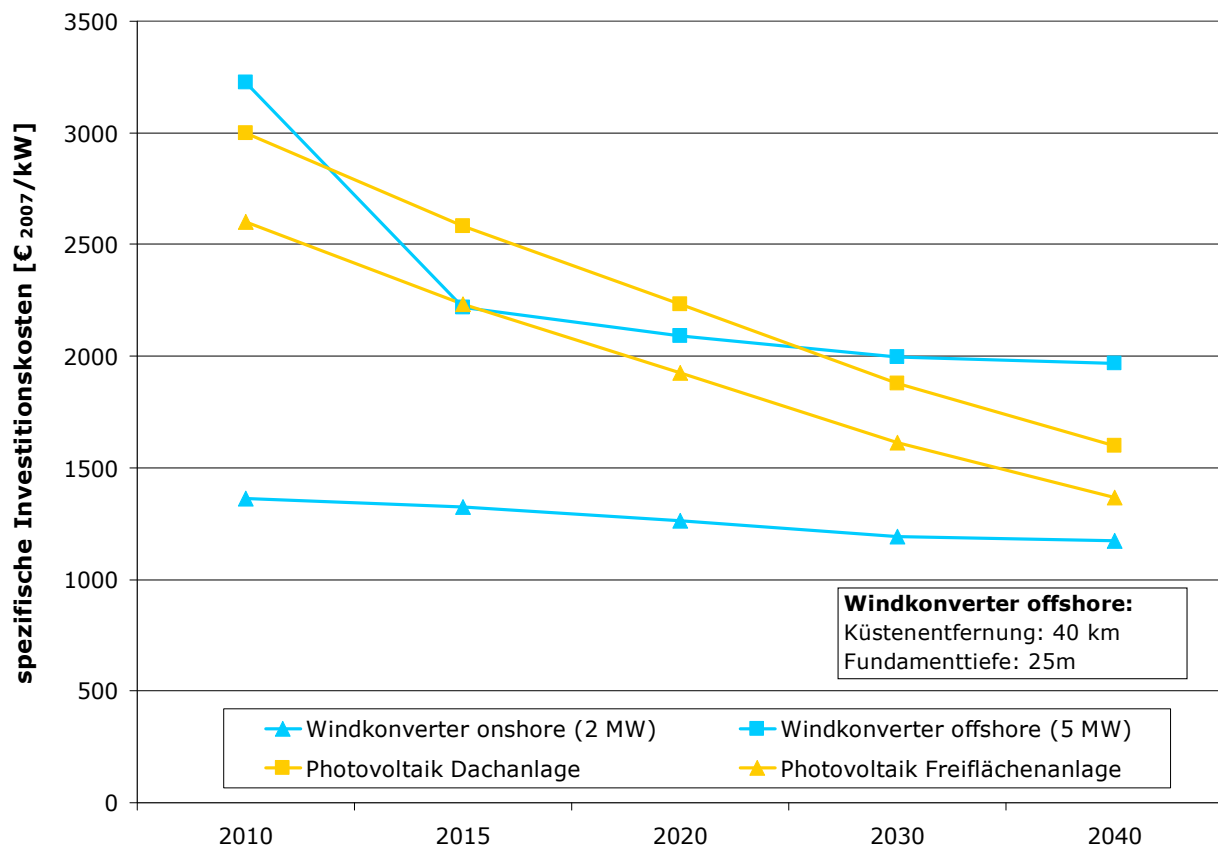
Abbildung 3.17: Entwicklung der Investitionskosten für Windenergiekonverter (WEA) und Photovoltaikanlagen (PV).
