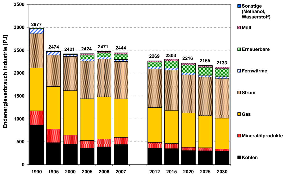
Abbildung 4.6: Endenergieverbrauch der Industrie nach Energieträgern in der Referenzprognose (Ra)
