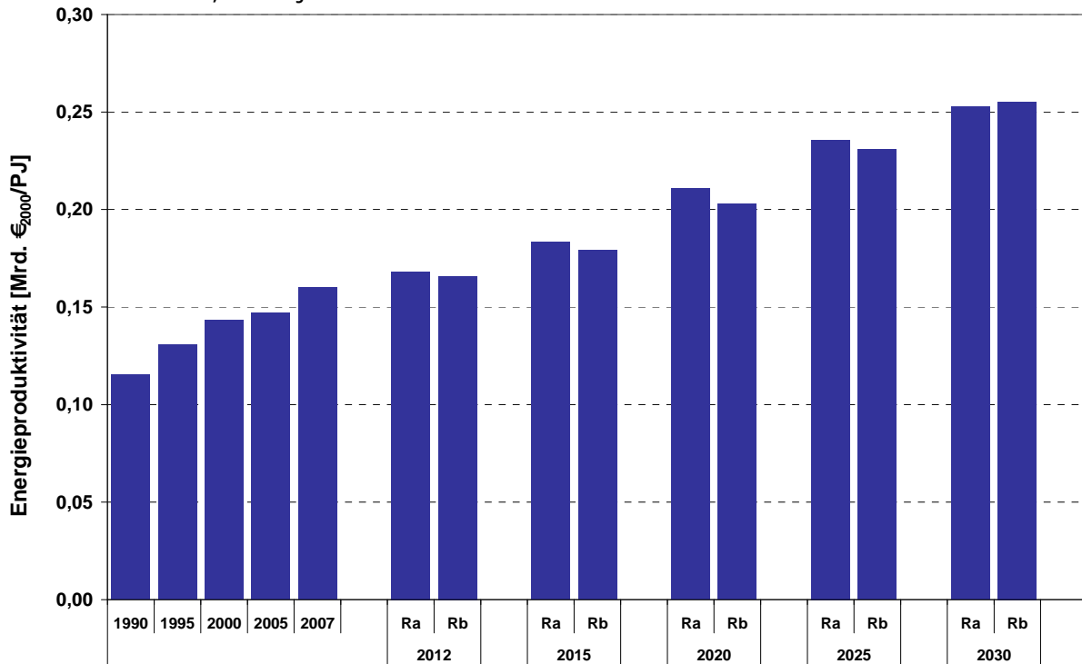
Abbildung 5.17: Energieproduktivität in der Referenzprognose (Ra) und in der Variante mit Laufzeitverlängerung (Rb)
