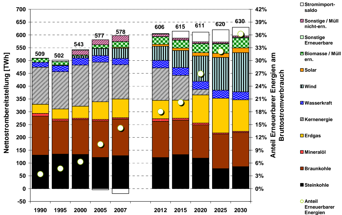
Abbildung 4.14: Nettostrombereitstellung in Deutschland in der Referenzprognose (Ra)
