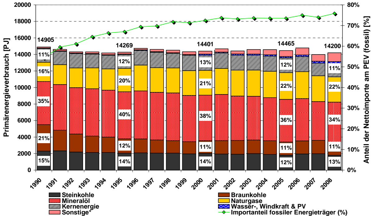
Abbildung 10.2: Primärenergieverbrauch nach Energieträgern in Deutschland
