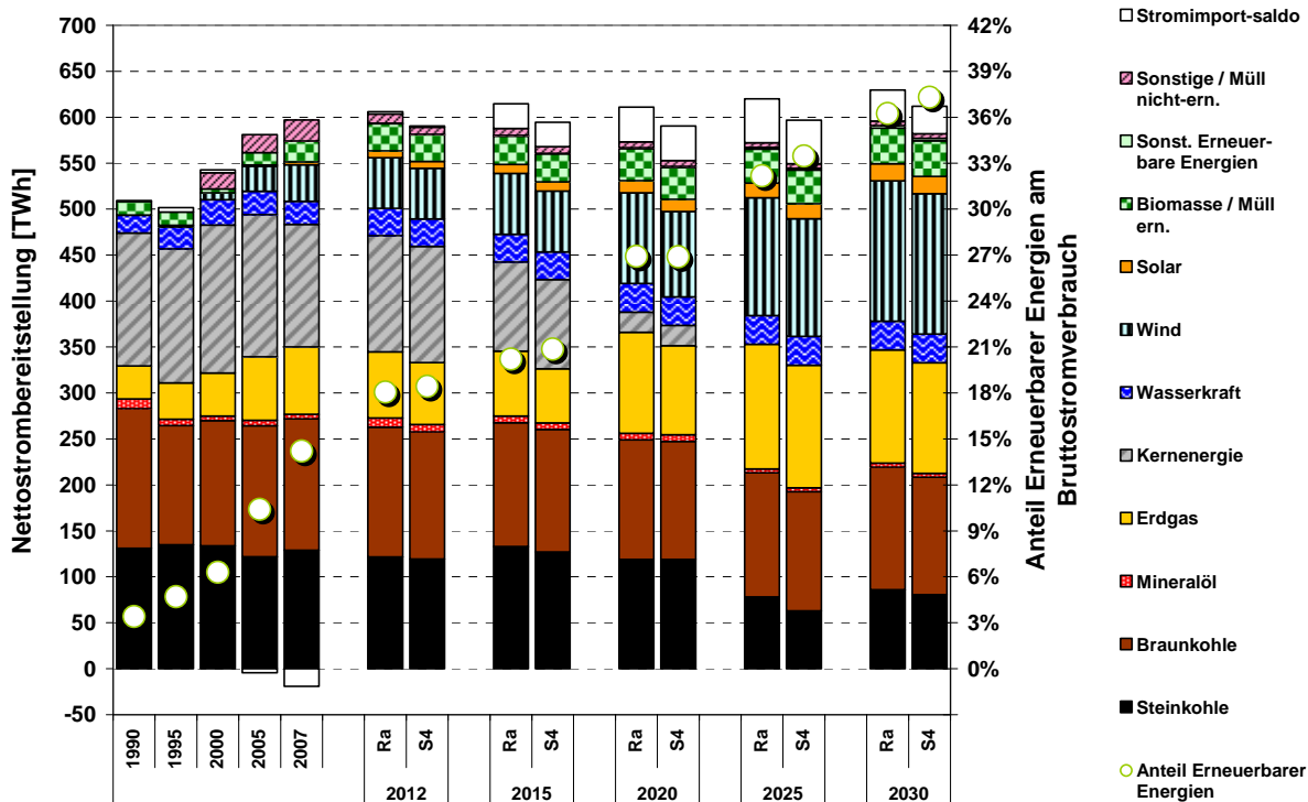
Abbildung 11.18: Nettostrombereitstellung in der Sensitivitätsanalyse „Niedrigere Bevölkerungsentwicklung“ (S4) im Vergleich zur Referenzprognose (Ra)
