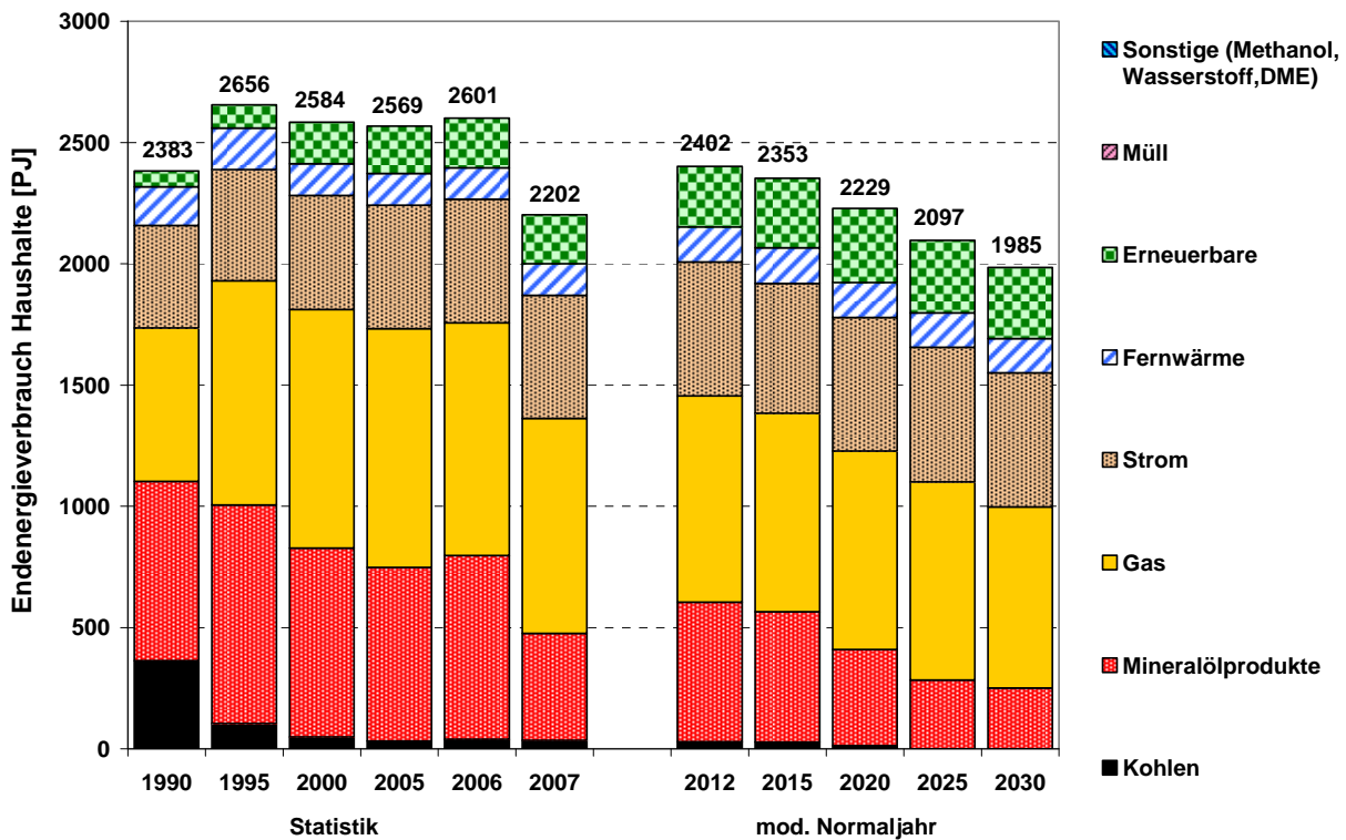
Abbildung 5.7: Entwicklung des Endenergieverbrauchs der Haushalte in der Variante mit Laufzeitverlängerung (Rb)
