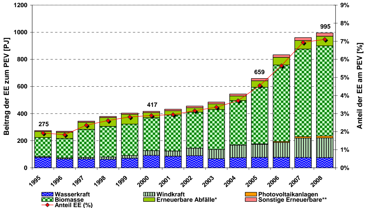
Abbildung 10.3: Beitrag der Erneuerbaren Energien zum Primärenergieverbrauch in Deutschland
