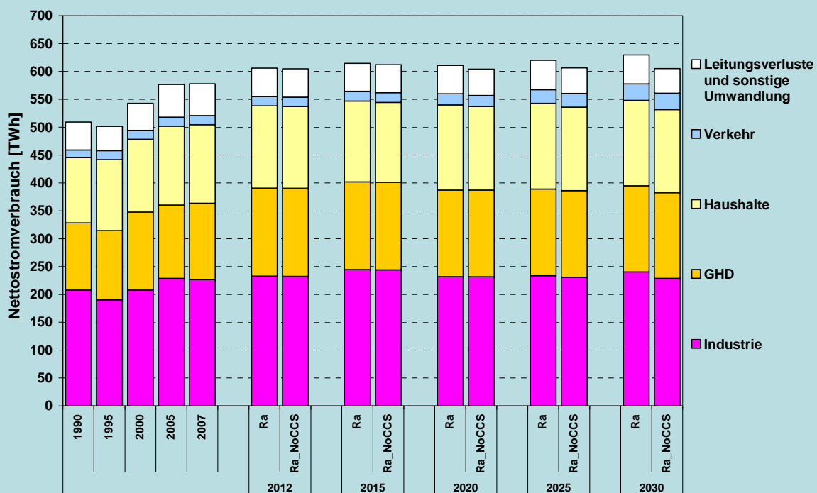
Abbildung 4.24: Nettostromverbrauch in der Referenzprognose (Ra) und in der Sensitivitätsanalyse „CCS wird nicht marktfähig“ (Ra_NoCCS)
