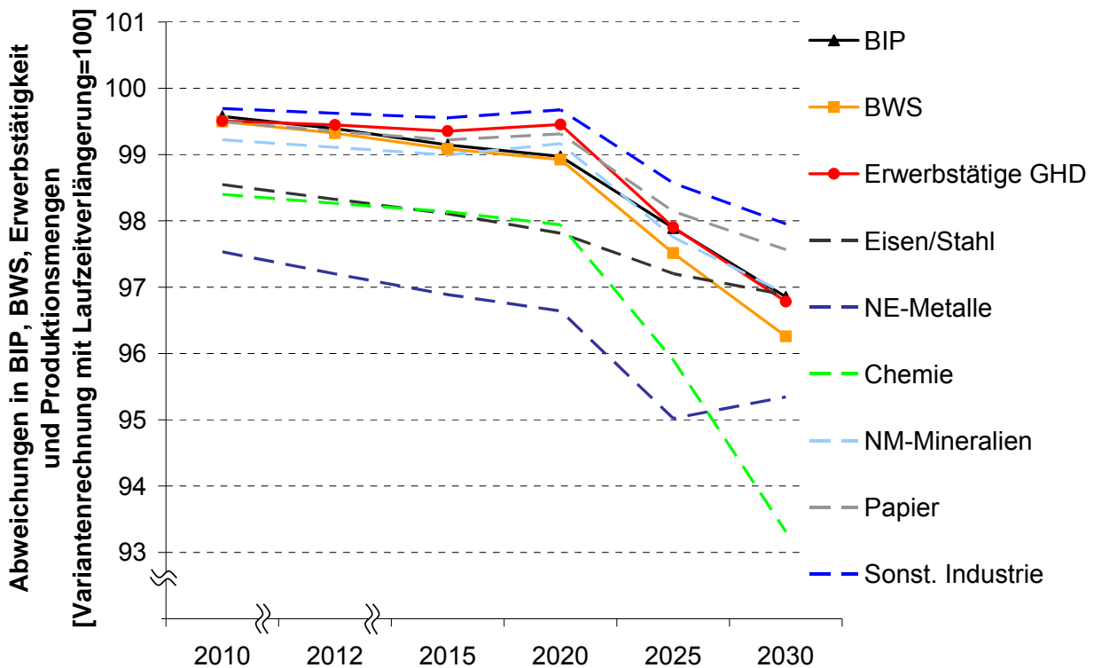
Abbildung 11.13: Veränderungen prognoserelevanter Inputgrößen in der Sensitivitätsanalyse „Verstärkter Klimaschutz bei Laufzeitverlängerung“ (S3d) gegenüber der Variante mit Laufzeitverlängerung (Rd)
