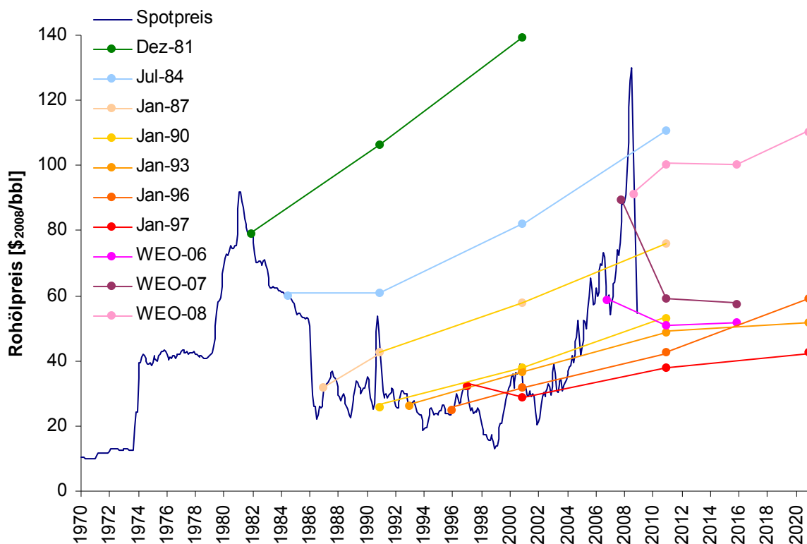
Abbildung 3.10: Verschiedene Ölpreisprognosen in realen Preisen (Schrattenholzer 1998, IEA2006, IEA 2007, IEA 2008d, EIA 2008)
