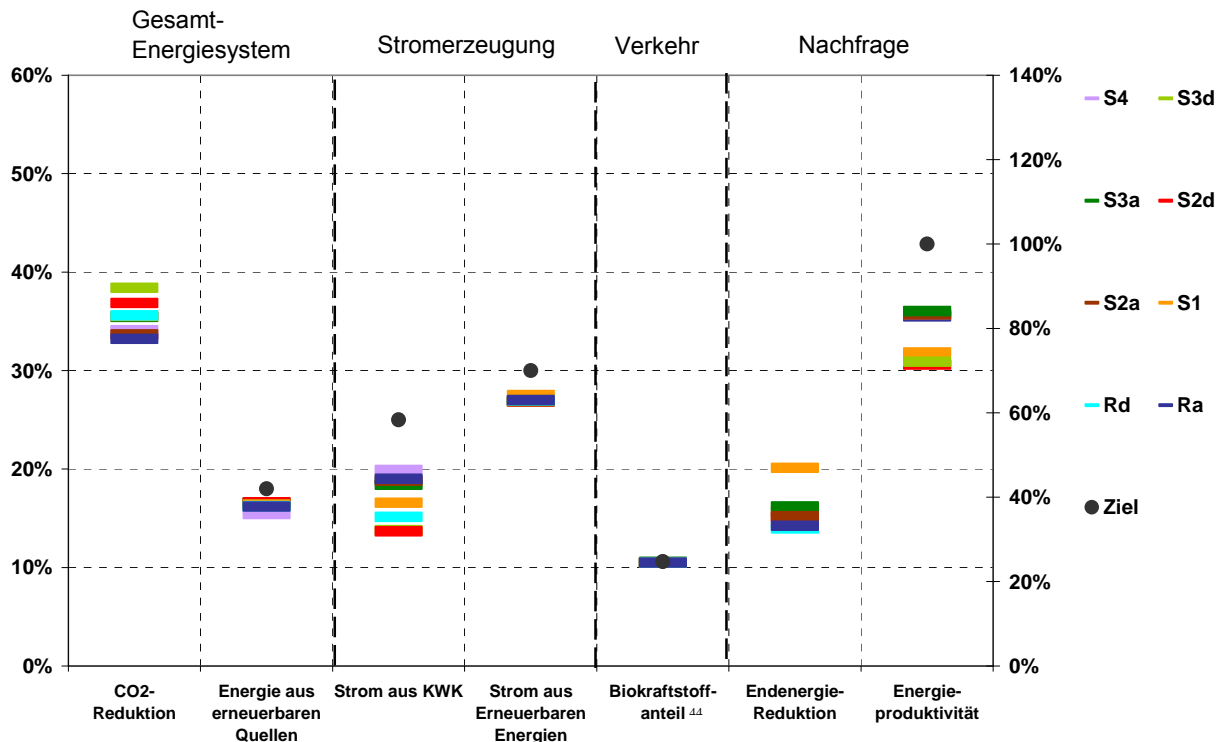
Abbildung 6.2: Erreichung energie- und klimapolitischer Ziele in den Sensitivitätsanalysen in 2020
