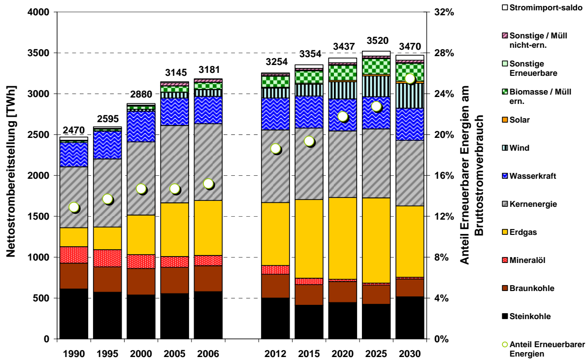
Abbildung 4.2: Nettostrombereitstellung in der EU-27 in der Referenzprognose (Ra)
