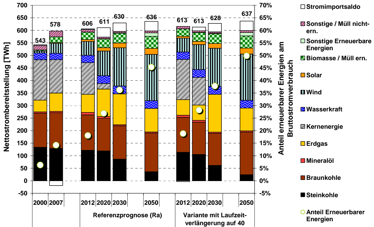
Abbildung 8.3: Ausblick 2050 zur Entwicklung der Nettostromerzeugung nach Energieträgern in Deutschland in der Referenzprognose (Ra) (links) und in der Variante mit Laufzeitverlängerung (Rb) (rechts)
