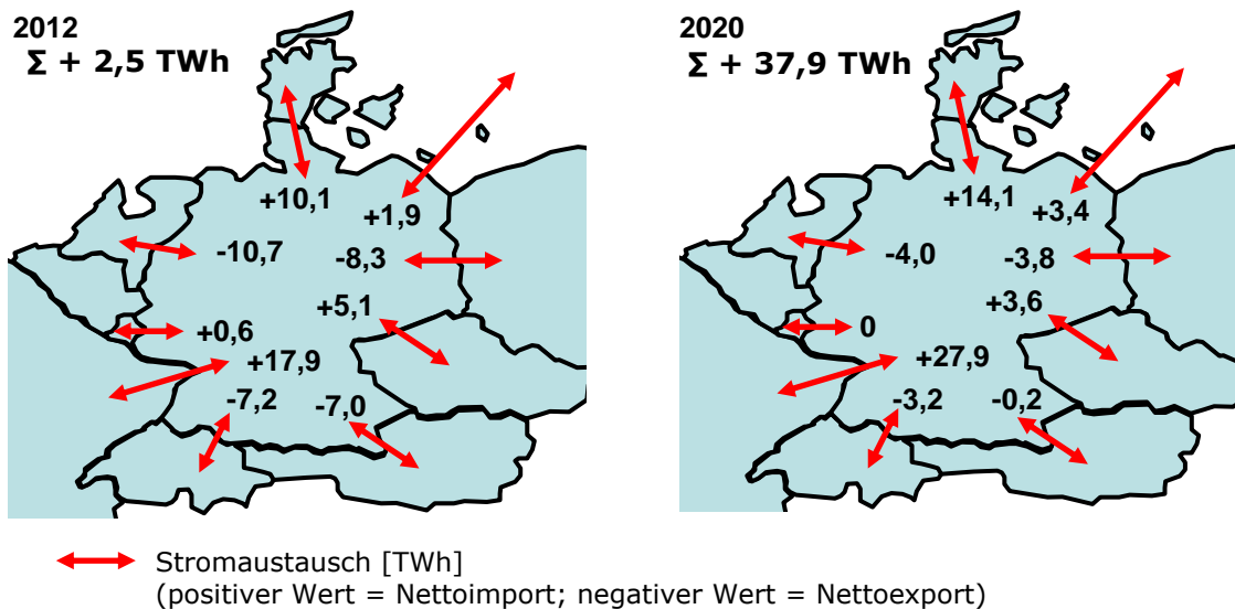
Abbildung 4.15: Stromimportsaldo Deutschlands in 2012 und 2020 in der Referenzprognose (Ra)
