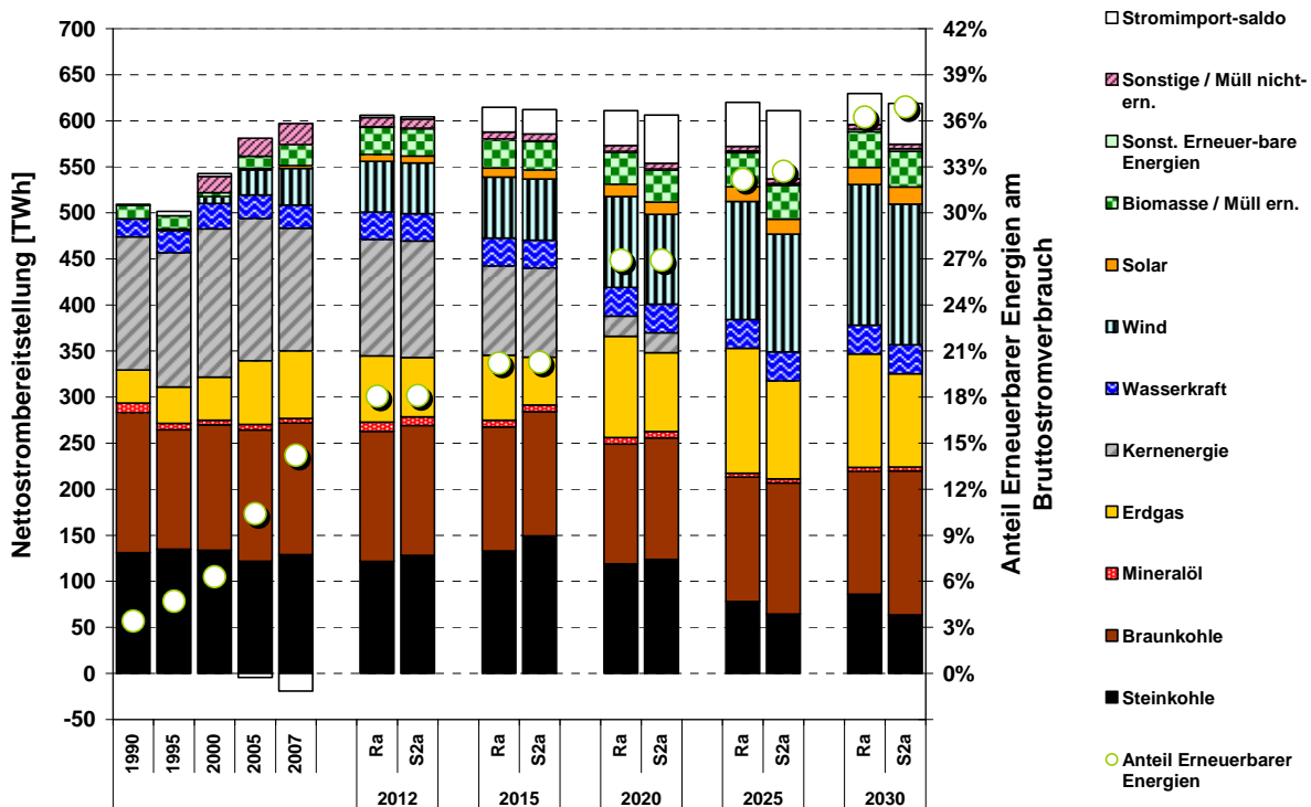
Abbildung 11.6: Nettostrombereitstellung in der Sensitivitätsanalyse „Hohe Ölpreise bei Kernenergieausstieg“ (S2a) im Vergleich zur Referenzprognose (Ra)
