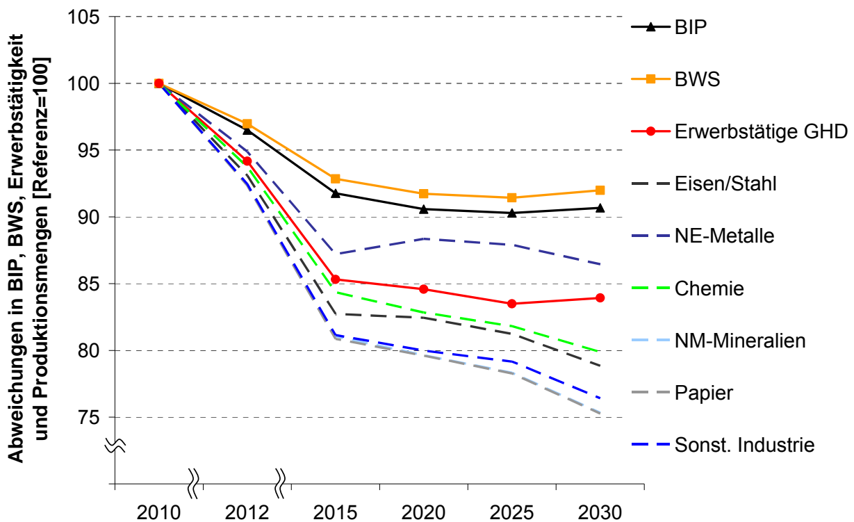
Abbildung 11.1: Veränderung prognoserelevanter Inputgrößen in der Sensitivitätsanalyse „Die Krise dauert länger“ (S1) gegenüber der Referenzprognose (Ra)
