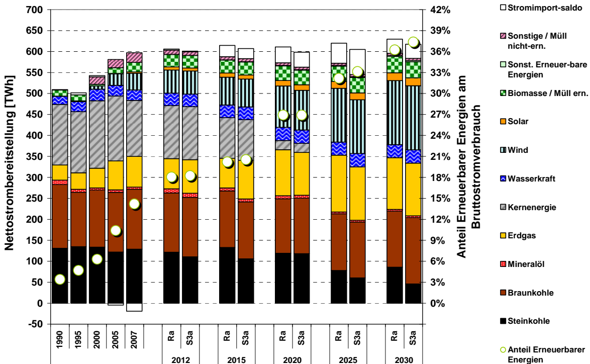
Abbildung 11.12: Nettostrombereitstellung in der Sensitivitätsanalyse „Verstärkter Klimaschutz bei Kernenergieausstieg“ (S3a) im Vergleich zur Referenzprognose (Ra)
