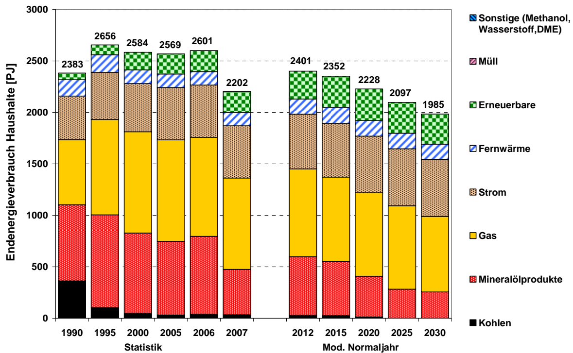
Abbildung 4.8: Entwicklung des Endenergieverbrauchs der Haushalte in der Referenzprognose (Ra)
