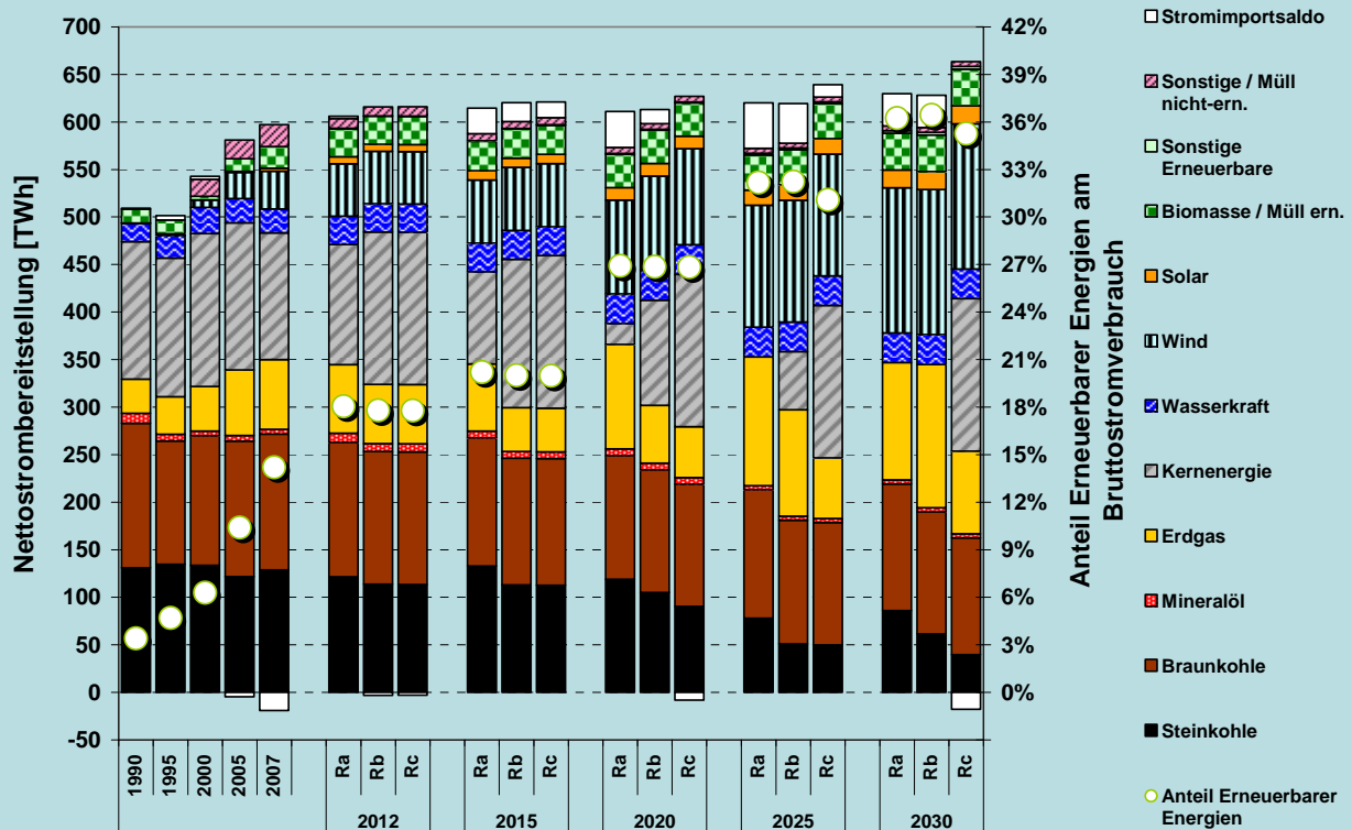
Abbildung 5.21: Nettostrombereitstellung in der Variante „Laufzeitverlängerung der Kernkraftwerke auf 60 Jahre“ (Rc) im Vergleich zur Referenzprognose (Ra) und zur Variante mit Laufzeitverlängerung auf 40 Jahre (Rb)
