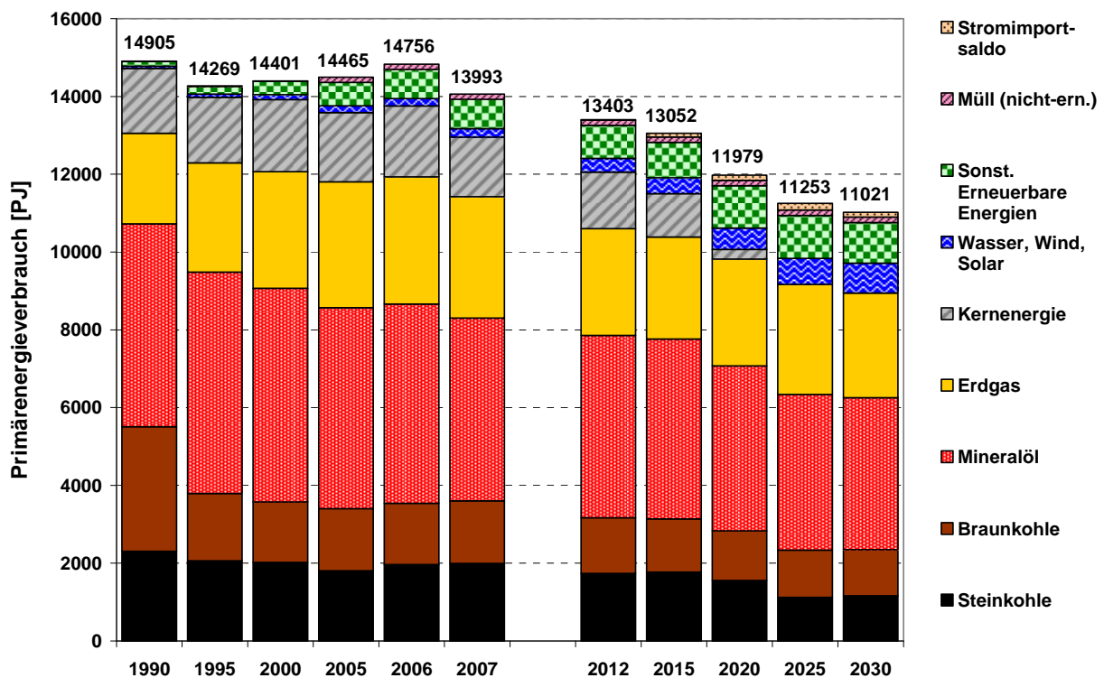
Abbildung 4.27: Primärenergieverbrauch in Deutschland nach Energieträgern in der Referenzprognose (Ra)
