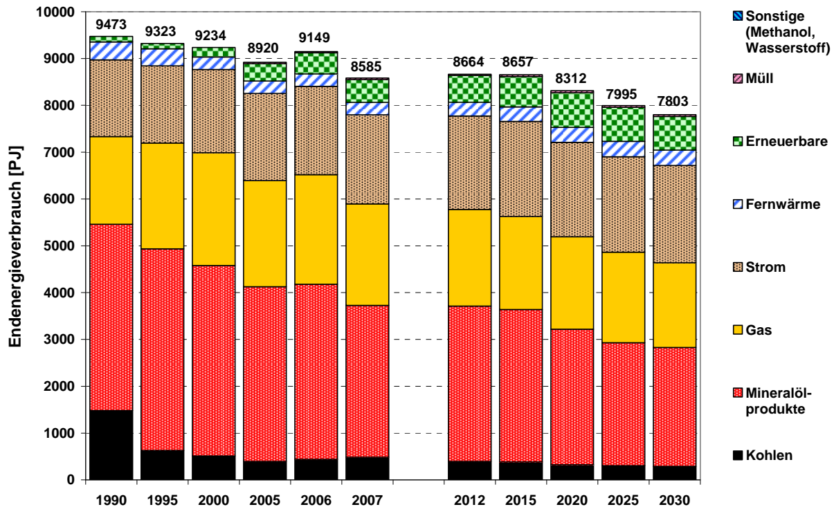
Abbildung 4.11: Endenergieverbrauch nach Energieträgern in der Referenzprognose (Ra)
