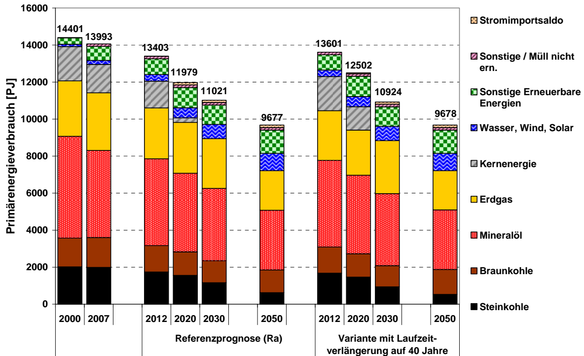
Abbildung 8.1: Ausblick 2050 zur Entwicklung des Primärenergieverbrauchs in der Referenzprognose (Ra) (links) und in der Variante mit Laufzeitverlängerung (Rb) (rechts)
