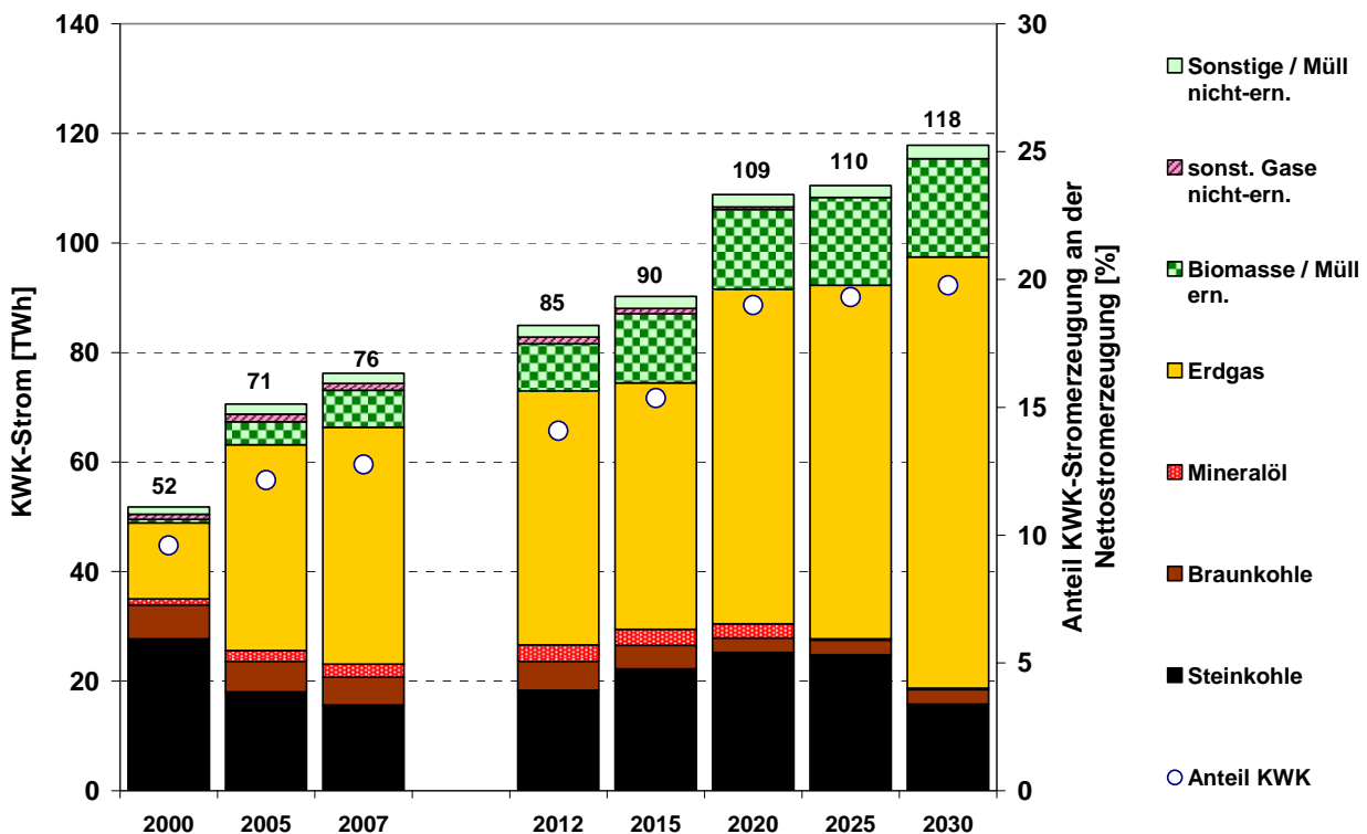
Abbildung 4.26: KWK-Stromerzeugung in der Referenzprognose (Ra)
