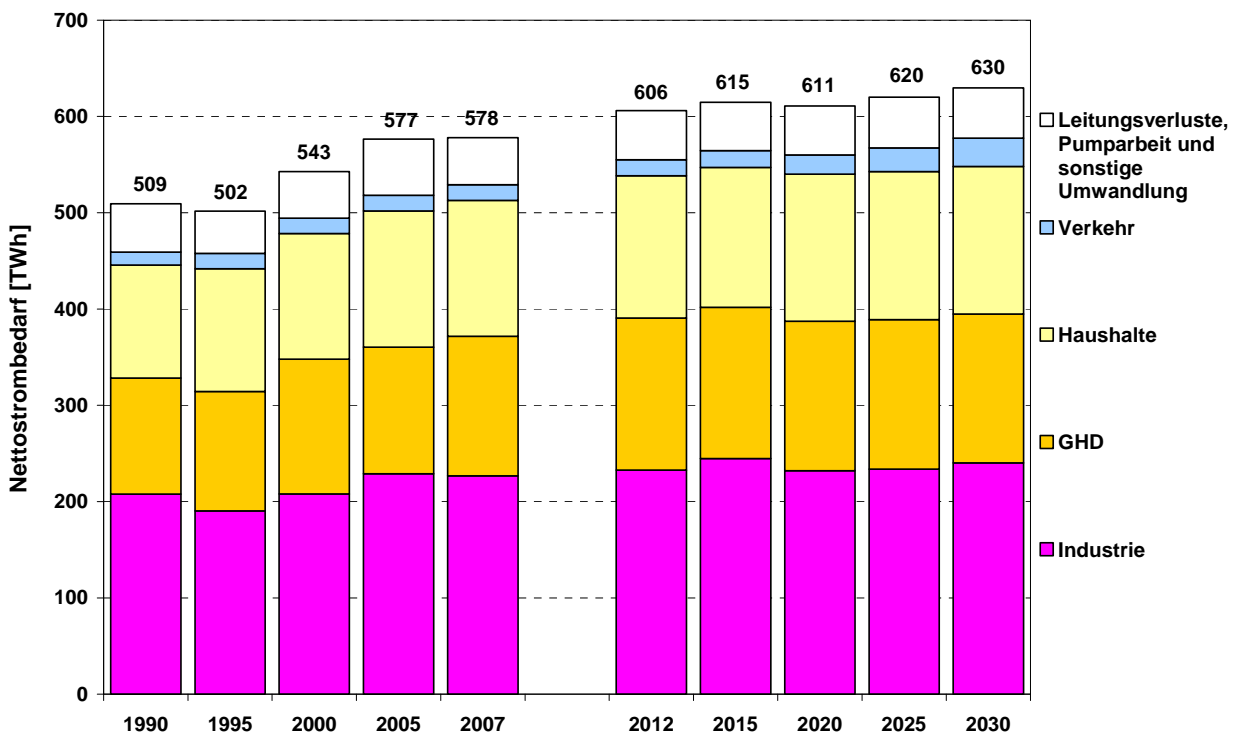
Abbildung 4.13: Nettostrombedarf in Deutschland in der Referenzprognose (Ra)
