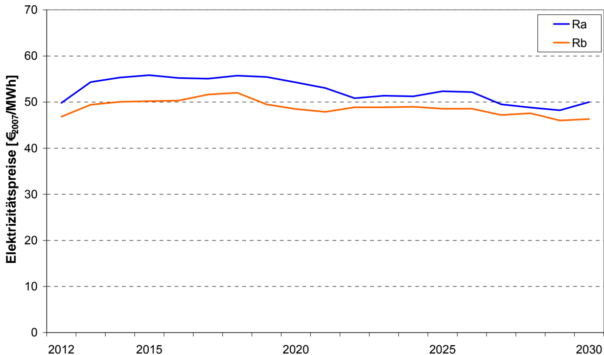
Abbildung 5.2: Jahresdurchschnittspreise für Elektrizität am deutschen Großhandelsmarkt in der Referenzprognose (Ra) und in der Variante mit Laufzeitverlängerung (Rb)
