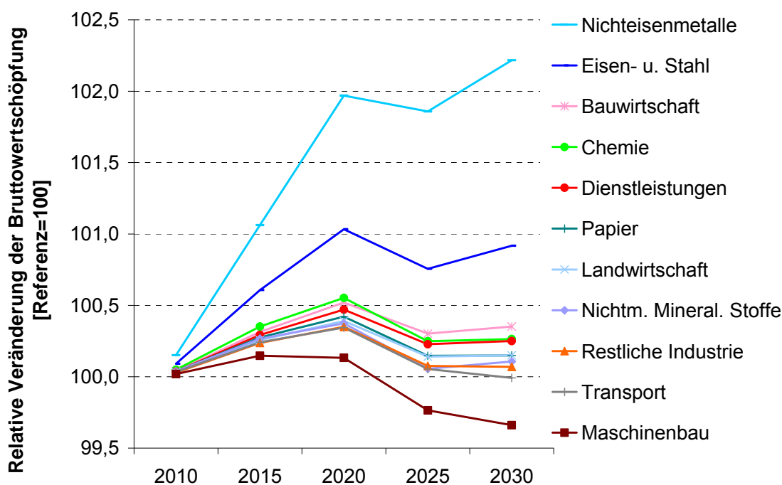
Abbildung 5.3: Wertschöpfungseffekte bei einer Laufzeitverlängerung der Kernkraftwerke
