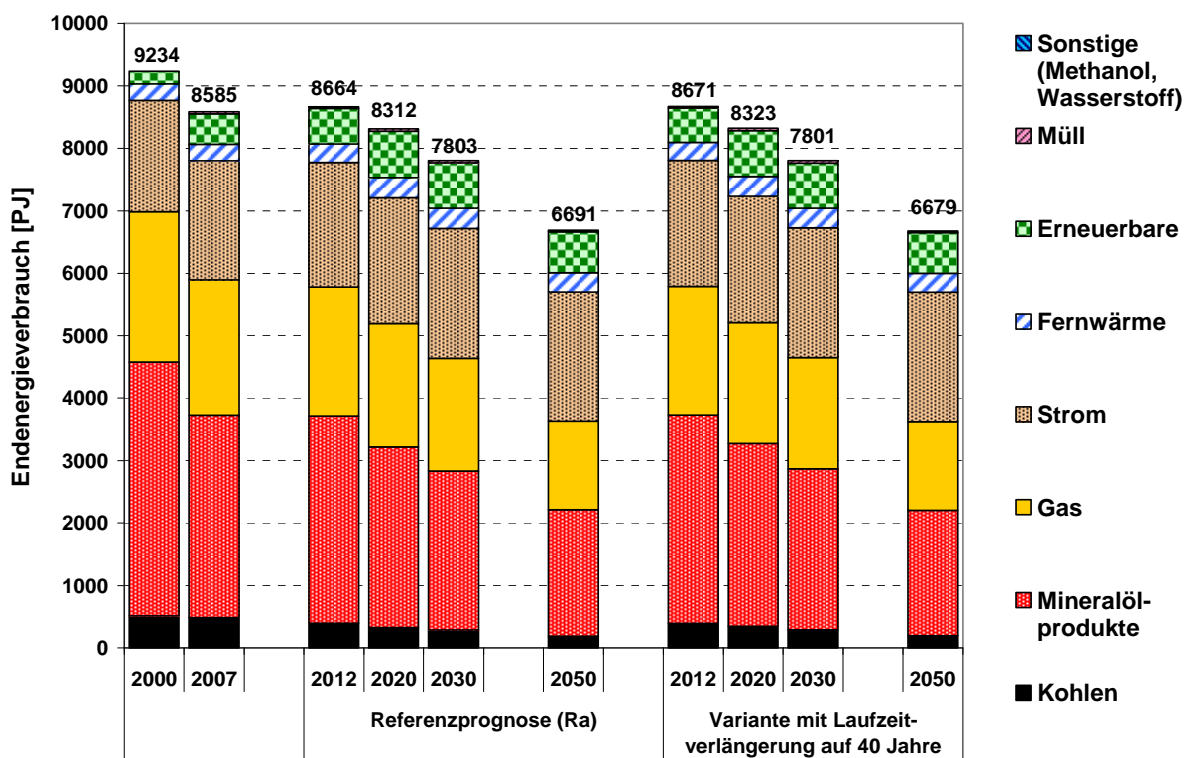
Abbildung 8.2: Ausblick 2050 zur Entwicklung des Endenergieverbrauchs in der Referenzprognose (Ra) (links) und in der Variante mit Laufzeitverlängerung (Rb) (rechts)
