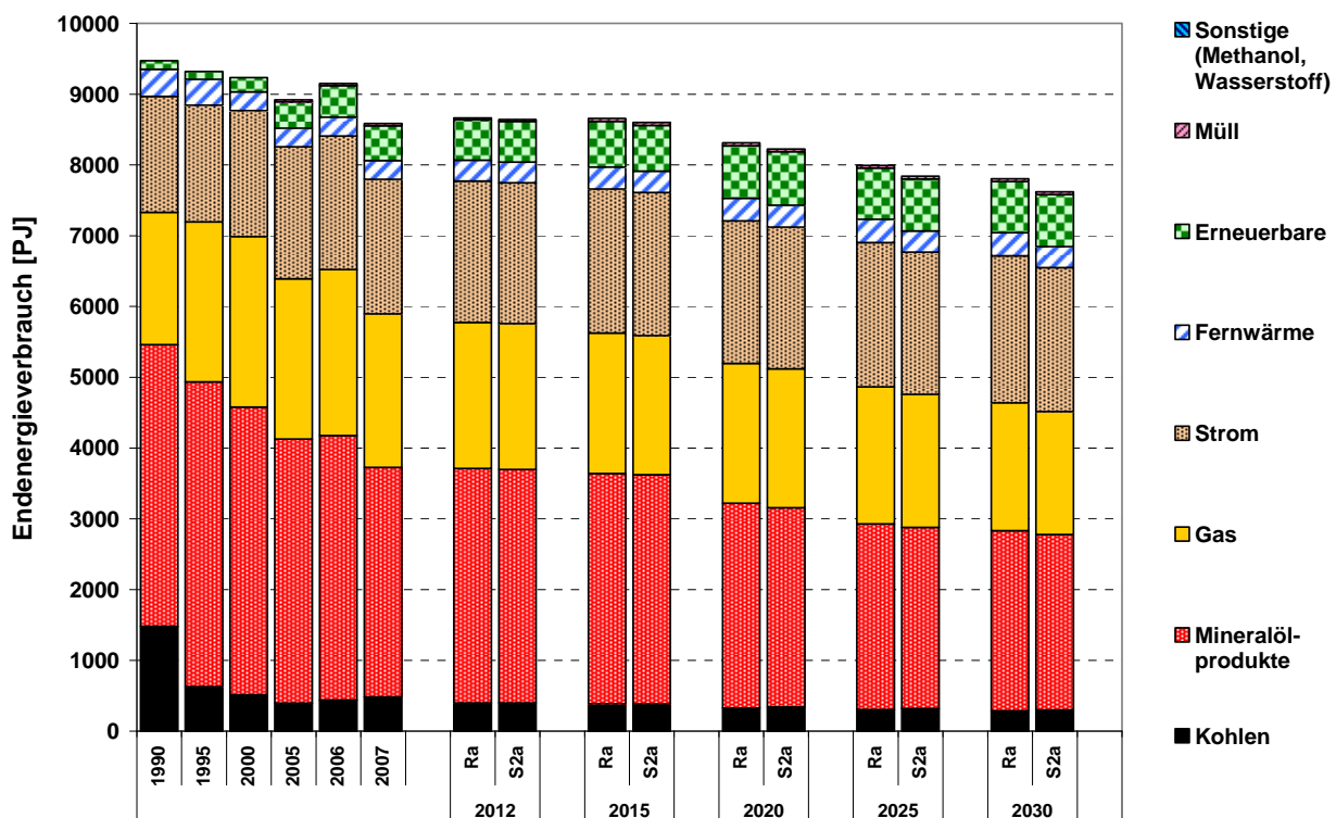
Abbildung 11.5: Endenergieverbrauch in der Sensitivitätsanalyse „Hohe Ölpreise bei Kernenergieausstieg“ (S2a) im Vergleich zur Referenzprognose (Ra)
