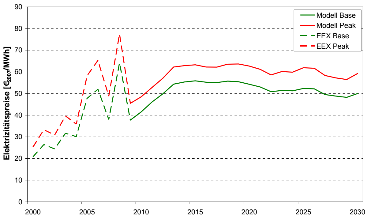
Abbildung 4.20: Reale Jahresdurchschnittspreise für Elektrizität am deutschen Großhandelsmarkt in der Referenzprognose (Ra)
