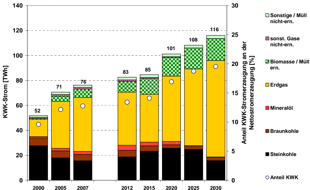
Abbildung 5.15: KWK-Stromerzeugung in der Variante mit Laufzeitverlängerung (Rb)
