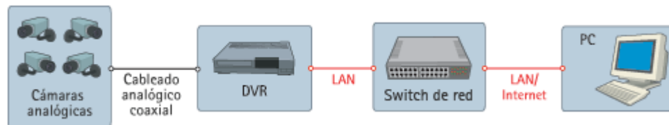
Figura 2: Diagrama de Sistema de CCTV Analógico con DVR Extraído de http://www.axis.com
