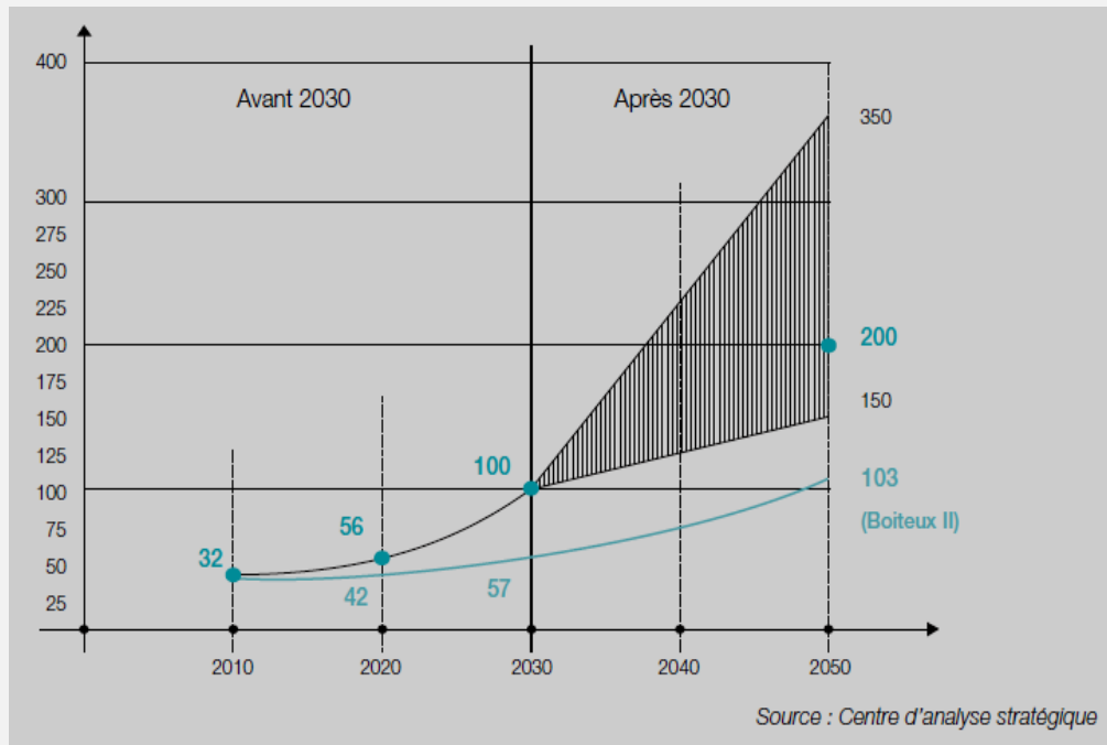
Figure 1. La valeur du CO 2 recommandée par la commission A. Quinet
