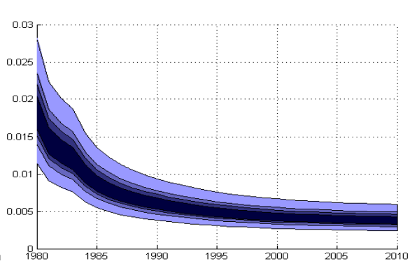
(d) Precision of beliefs (expectations)
