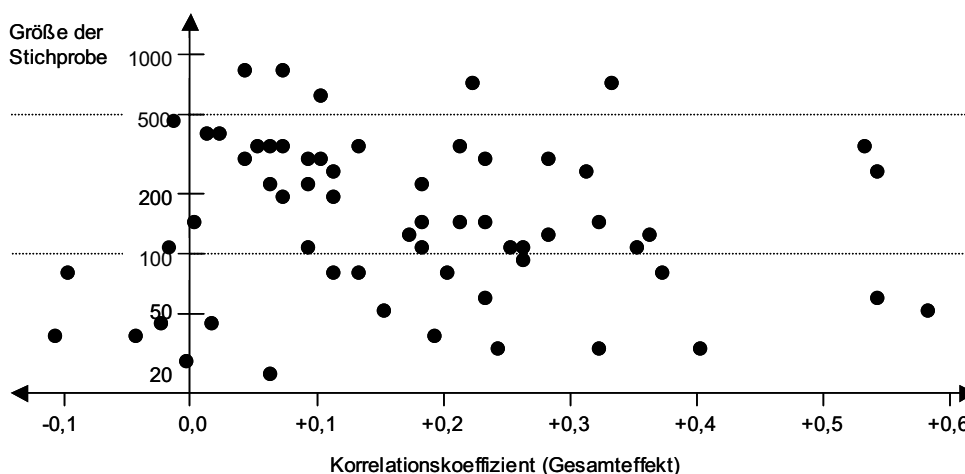
Abb. 3: Streudiagramm der Korrelationskoeffizienten aus den Primärstudien (Gesamteffekte)
