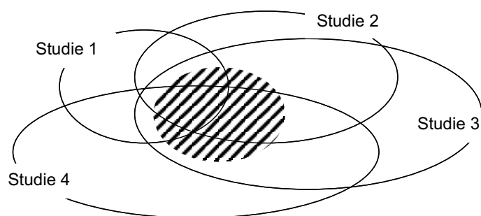
Abb. 1: Basisannahmen der Metaanalyse
