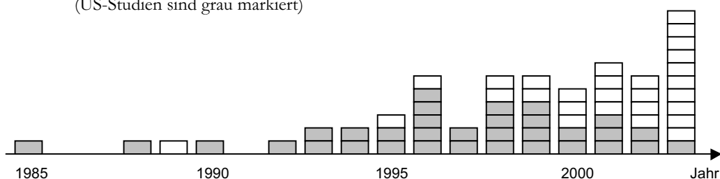
Abb. 2: Veröffentlichungsdatum der 61 Primärstudien (US-Studien sind grau markiert)
