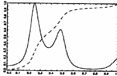
EURO15 GDP-Cycle
