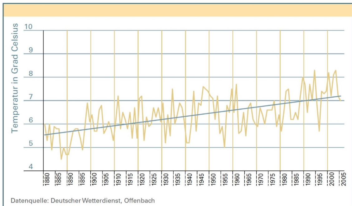
Abb. 3: Jahresmittel der Temperatur an der Messstation Hohenpeißenberg (1879–2005)
