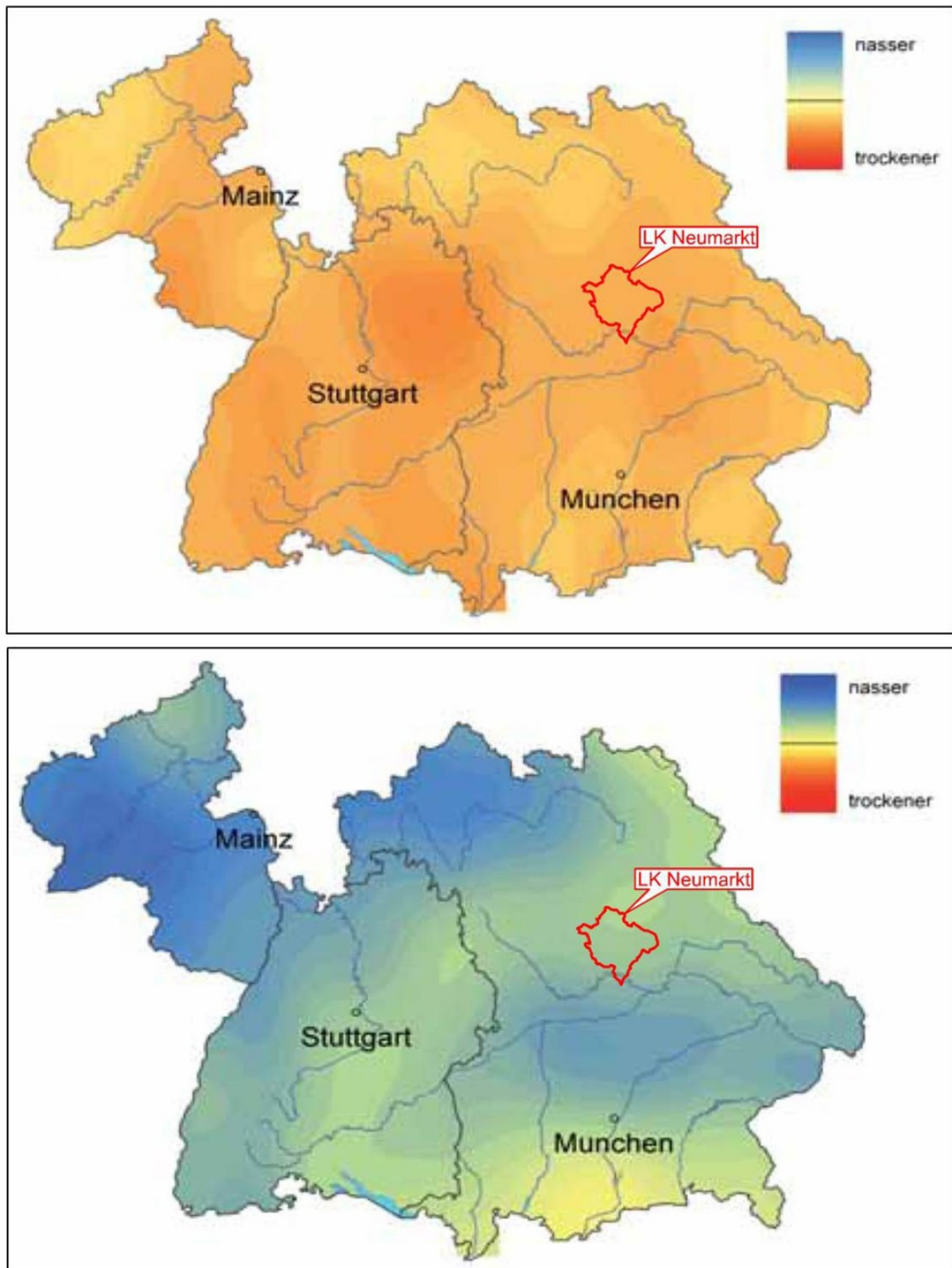
Abb. 5: Änderung der Sommer- (oben) und Winterniederschläge (unten) im Zeitraum 2021–2050 gegenüber 1971–2000 (ECHAM 5, WETTREG_2006)
