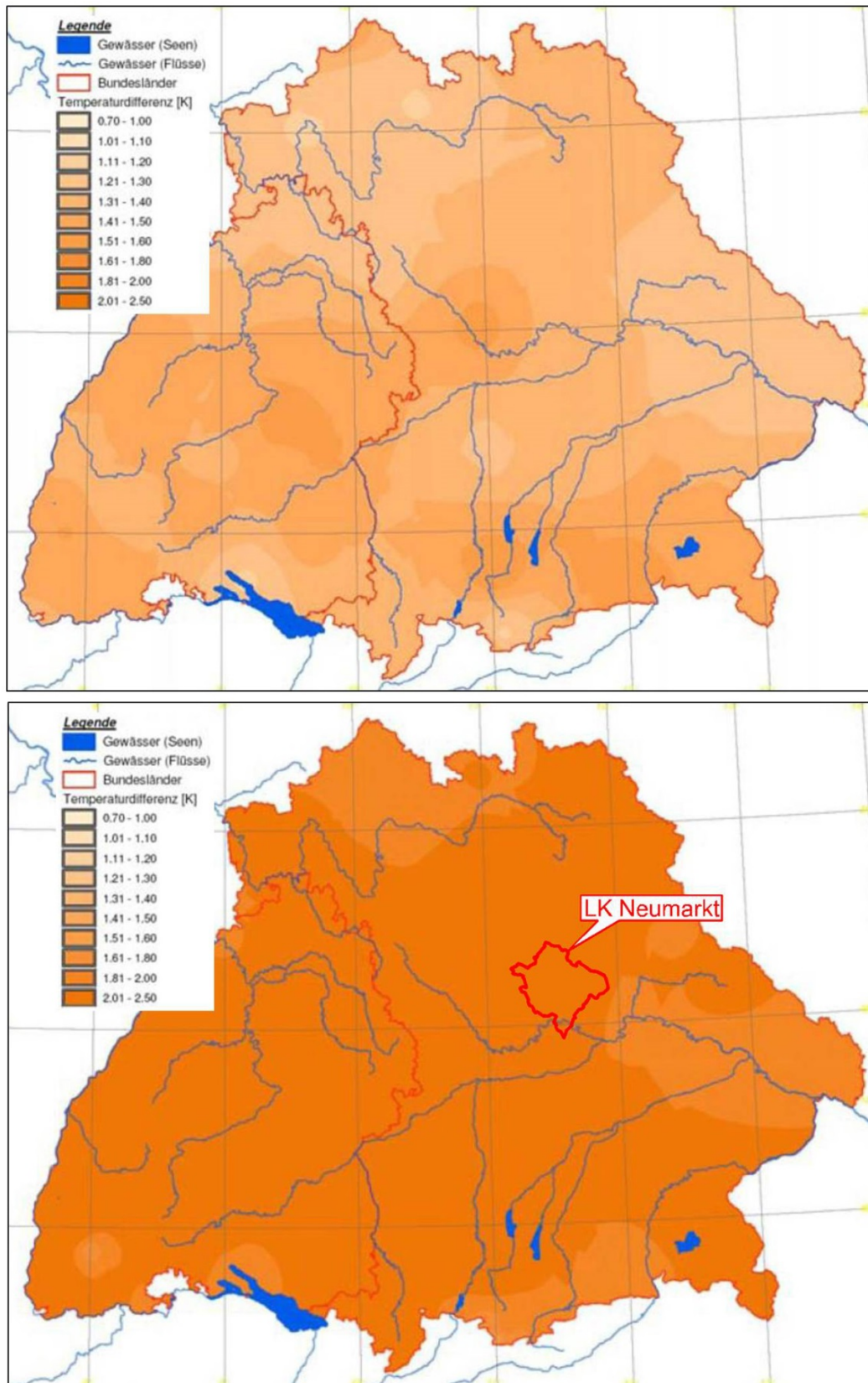
Abb. 4: Änderung der Sommer- (oben) und Wintertemperaturen (unten) im Zeitraum 2021–2050 gegenüber 1971–2000 (ECHAM 4, WETTREG_2003)
