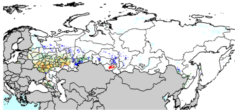
CSIRO-MK3 GCM
