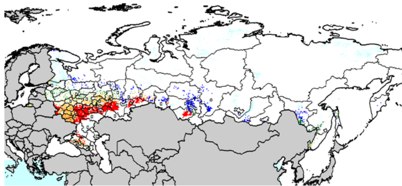
CNRM-CM3 GCM
