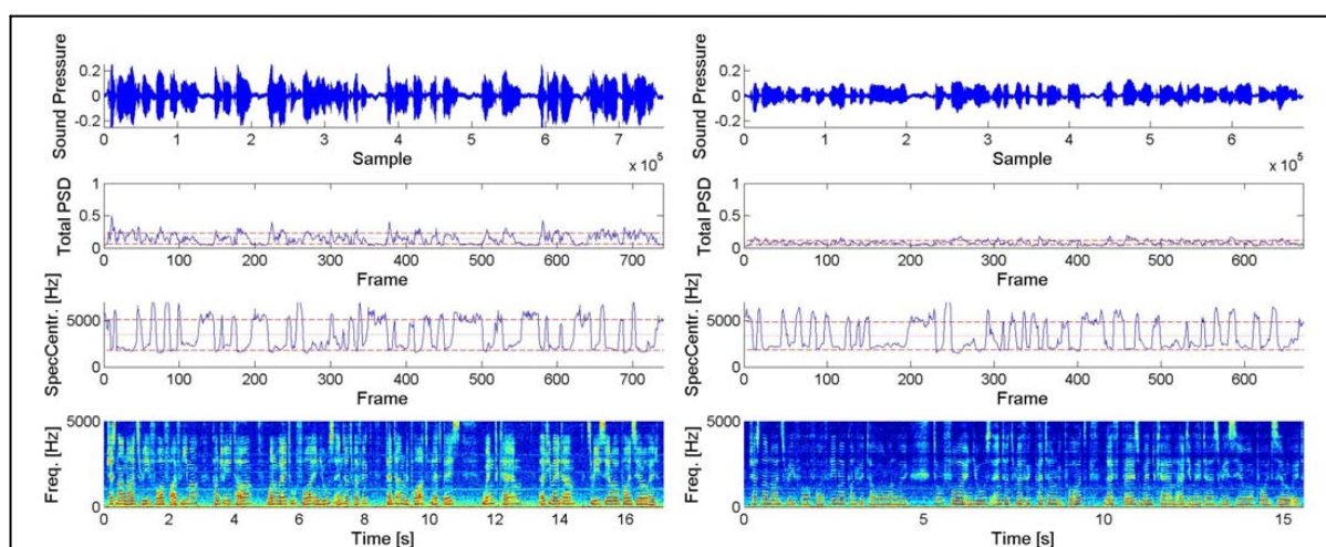
Abbildung 3: Spektrogramm zweier Stimmproben. Links ein selbstsicherer Sprecher und rechts ein unsicherer Sprecher. Dargestellt sind von oben nach unten Sound Pressure, Total Power Spectral Density (TPSD), Spectral Centroid (SpecCentr) und ein Spektrogramm. Hohe spektrale Leistungsdichten sind rot (im Schwarz-Weiß Druck: schwarz), niedrige hingegen blau (im Schwarz-Weiß Druck: grauwertig) kodiert.
