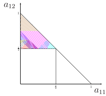
Feasible sets \mathcal{S}_{\mathcal{B}_1}-\mathcal{S}_{\mathcal{B}_7}
