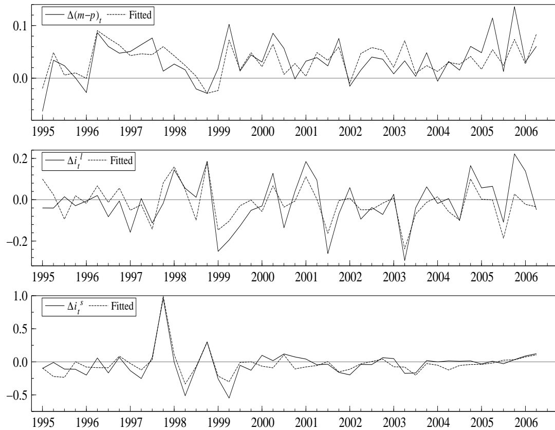
Figure 5: VECM: Actual and fitted values
